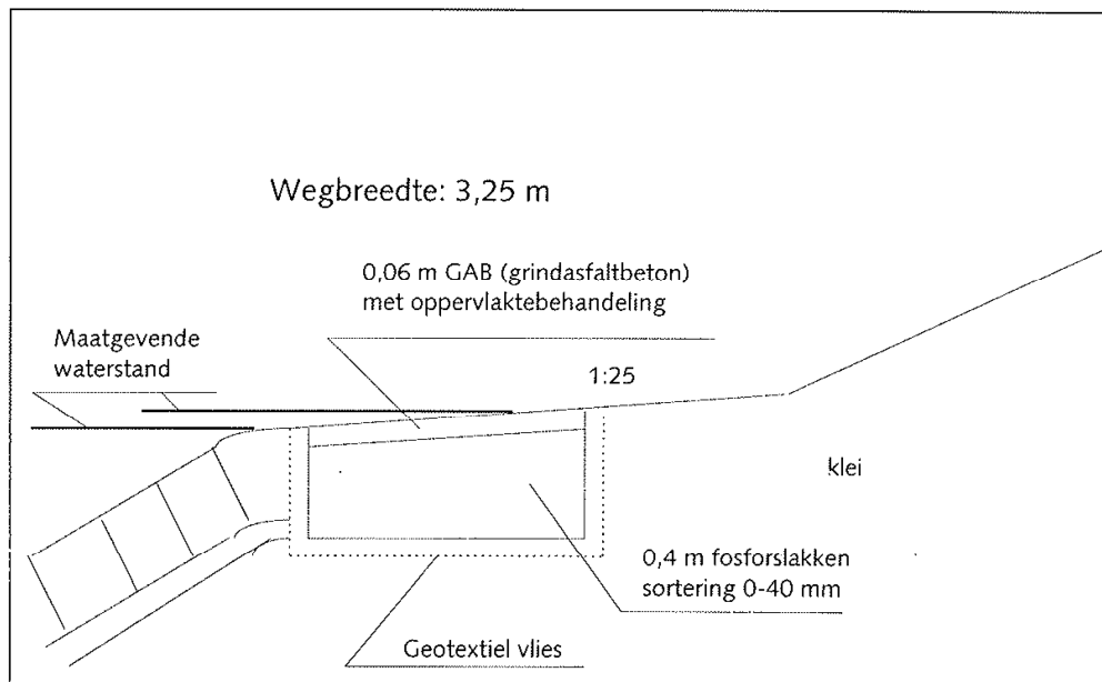
Figuur 2-1 Prinschesets van een onderhoudsstrook [Johanson, 2000]
