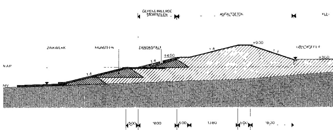
Figuur 0-22 Werkeiland Noordland en de bouwput [DBD, 1964]
