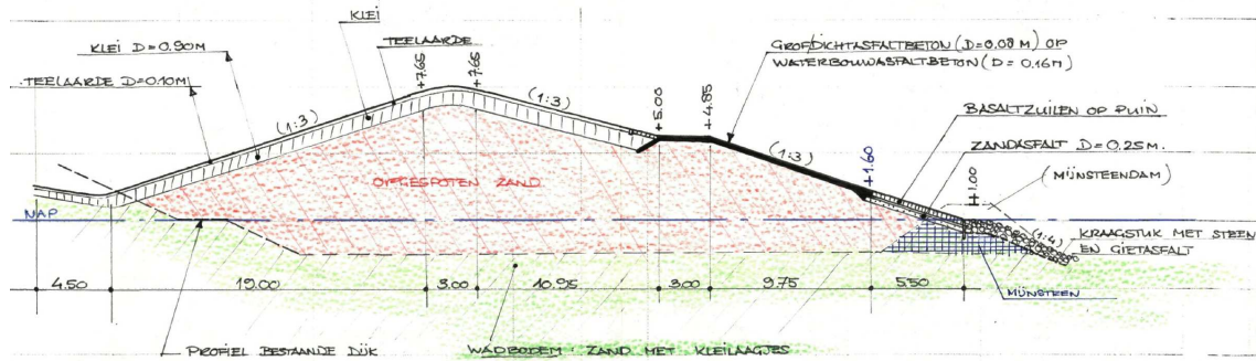
Figuur 0-37 Rijkzeeeewering Oude Schild [Thije, 1985]
