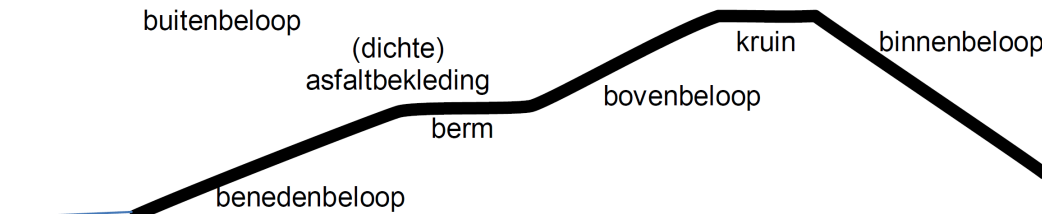
Figuur 3-1 A. Waterkering geheel bekleed met dichte bekledingen
