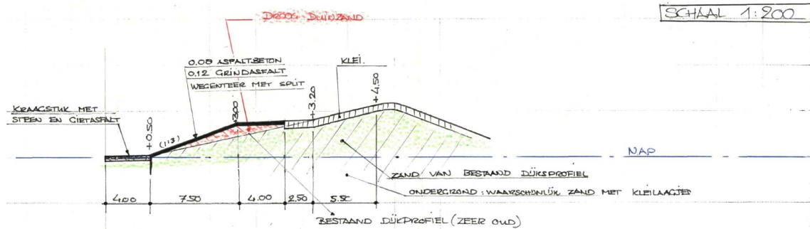
Figuur 0-39 Bolwerk Robbengat [Thije, 1985]
