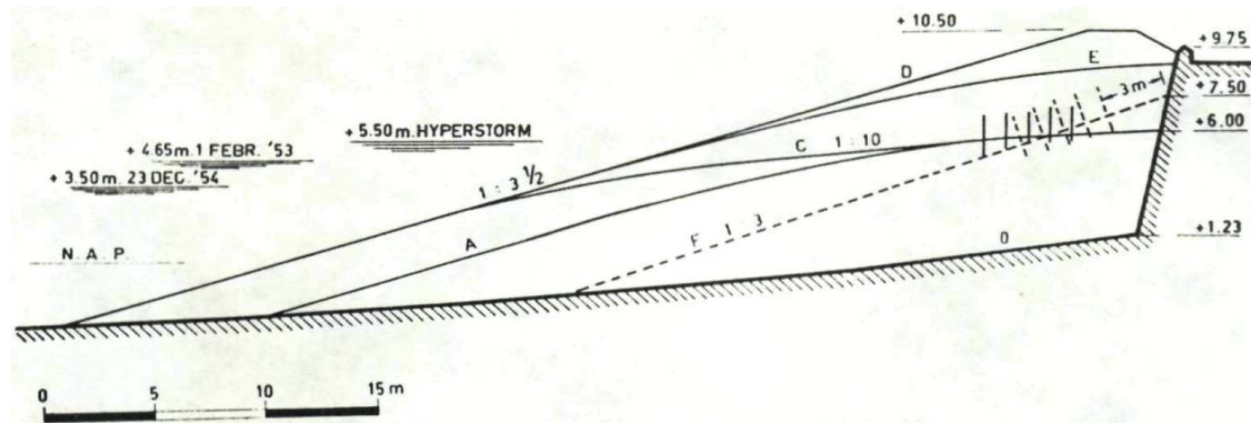
Figuur 2-4 Resultaten beproeving van verschillende bermprofielen in de windgoot t.b.v. boulevard de Ruyter
