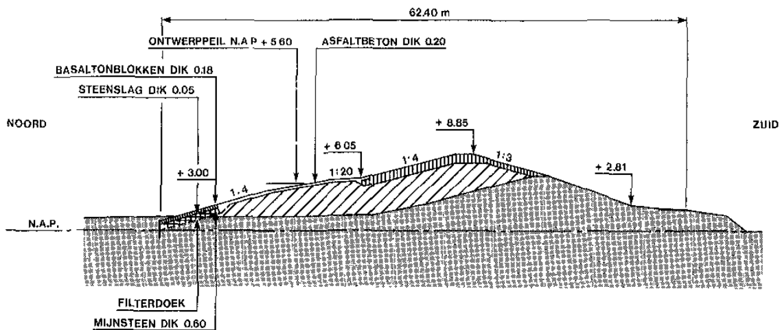
Figuur 0-25 Dwarsprofiel Ommelanderzeedijk [DBD, 1985]
