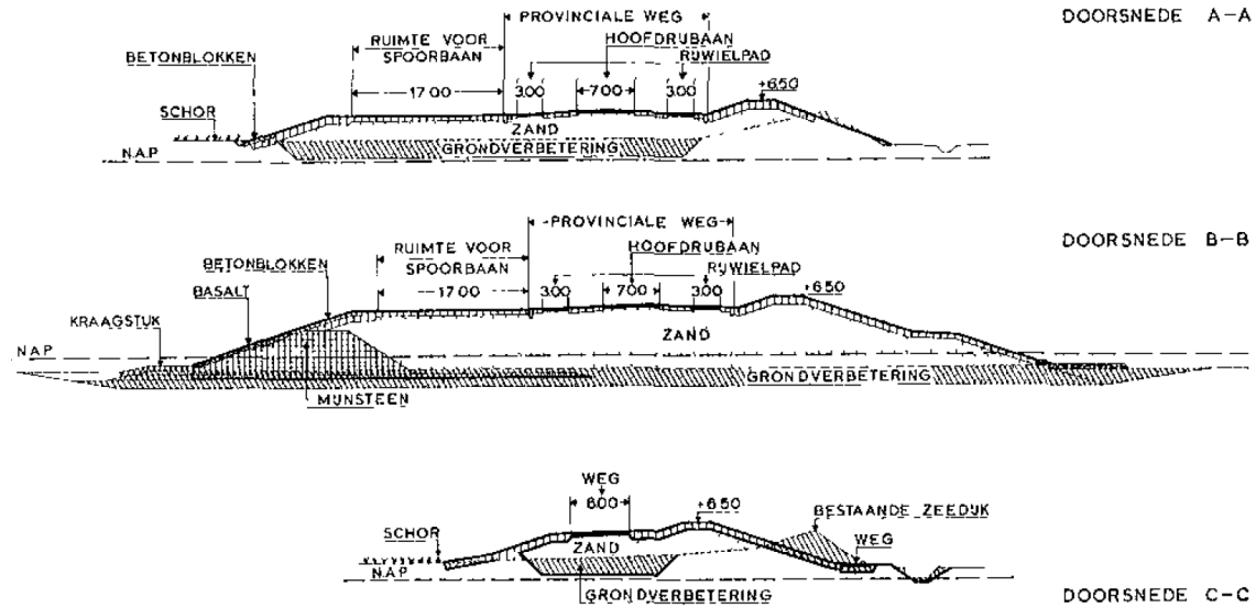
Figuur 0-15 Dwarsprofielen van de dijk rond het Zuider Sloe [DBD, 1962]
