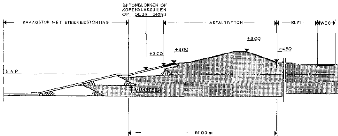
DOORSNEDE A Figuur 0-27 Plattegrond en doorsnede van het werkeiland op de Roggeplaat [DBD. 1969]
