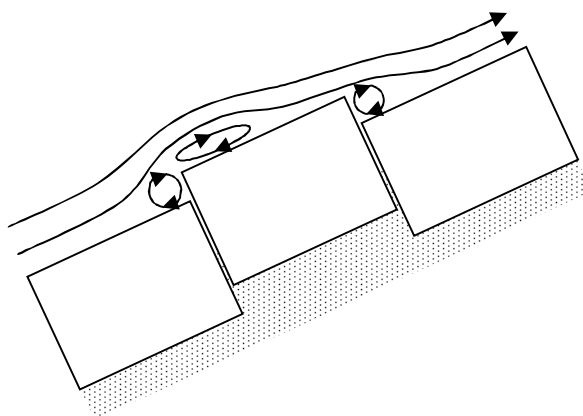
Figuur 6.1 Gekromde stroomlijnen over een uitstekende steen
