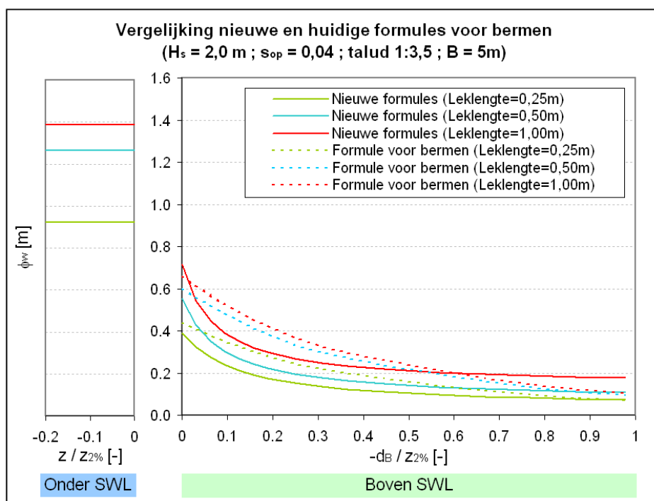
Figuur 6.9 Vergelijking nieuwe formules (5.3) en (5.4) en huidige formule voor bermen.
