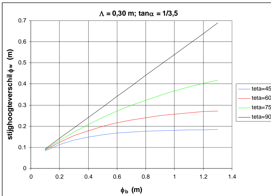
Figuur 5.5 Stijghoogteverschil als functie van \phi_b en \theta_r (teta) bij een leklengte van 0,3 m en een talud van 1:3,5.
