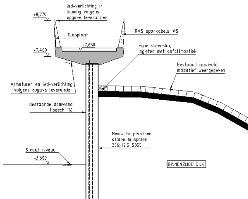
Figuur 4.1 Principe doorsnede keermuur
