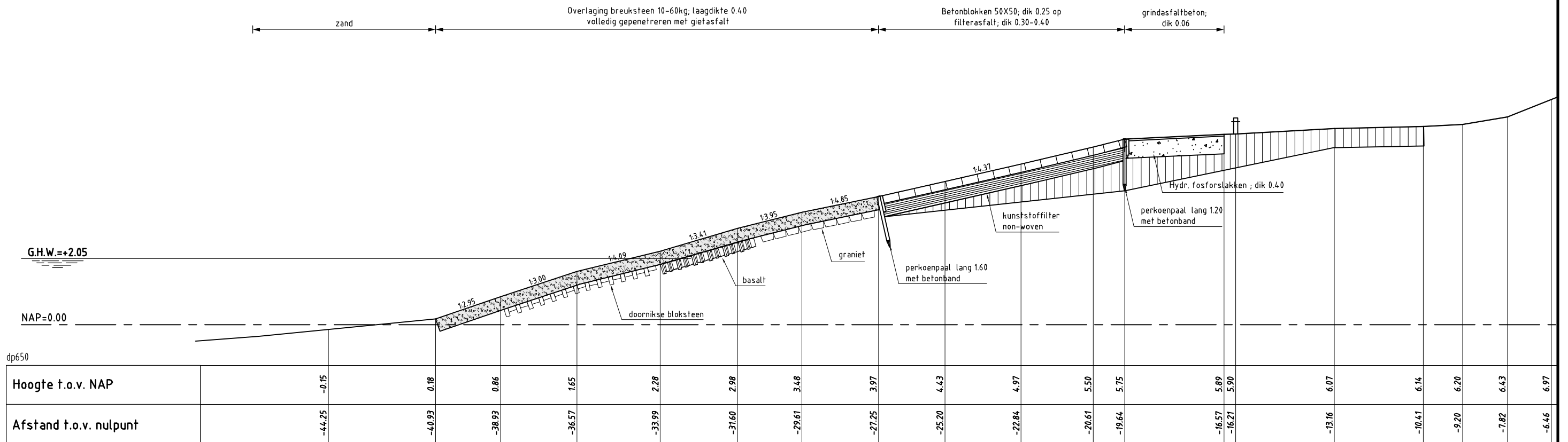
DWARSPROFIEL 6c bestaand
