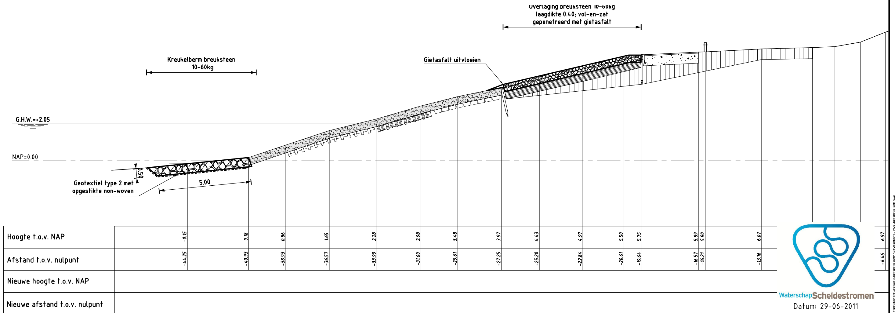
DWARSPROFIEL 6c nieuw
