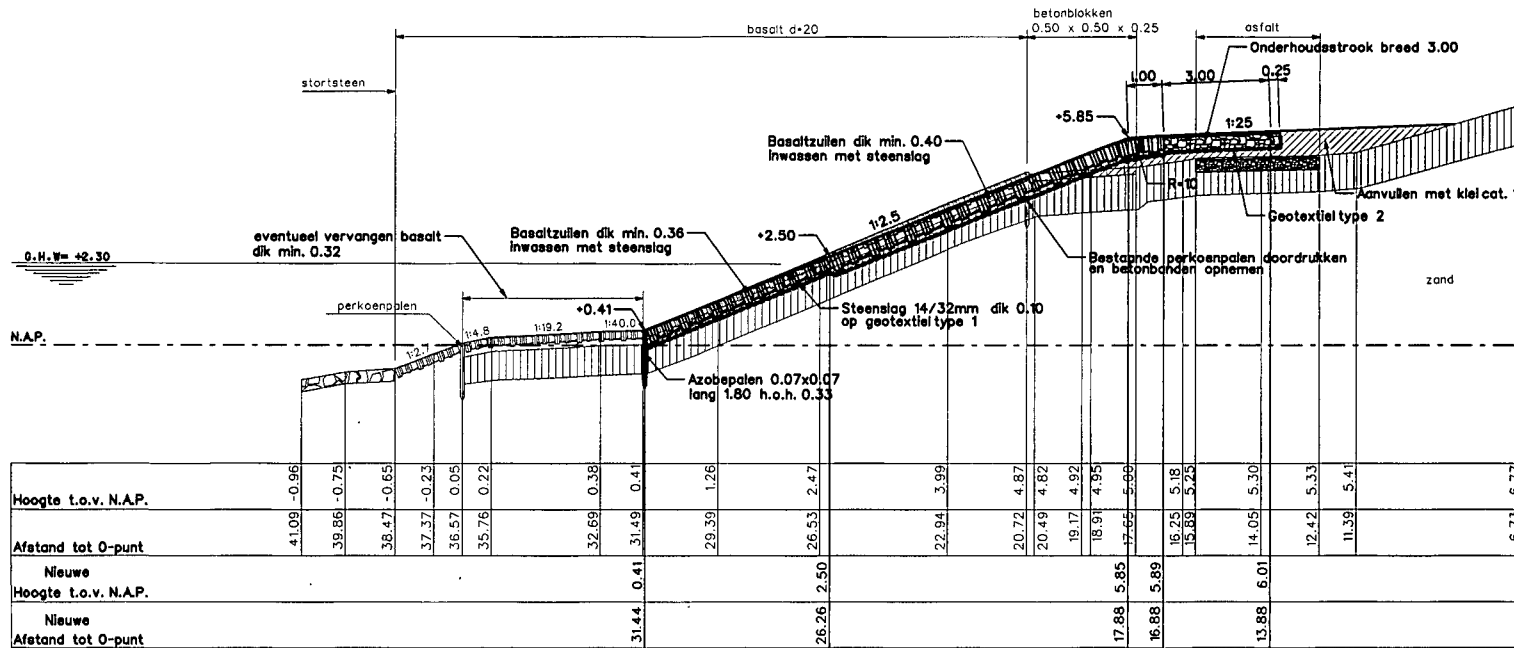
Dwarsprofiel 1 nieuw van dp84+15m tot circa dp84+60m
