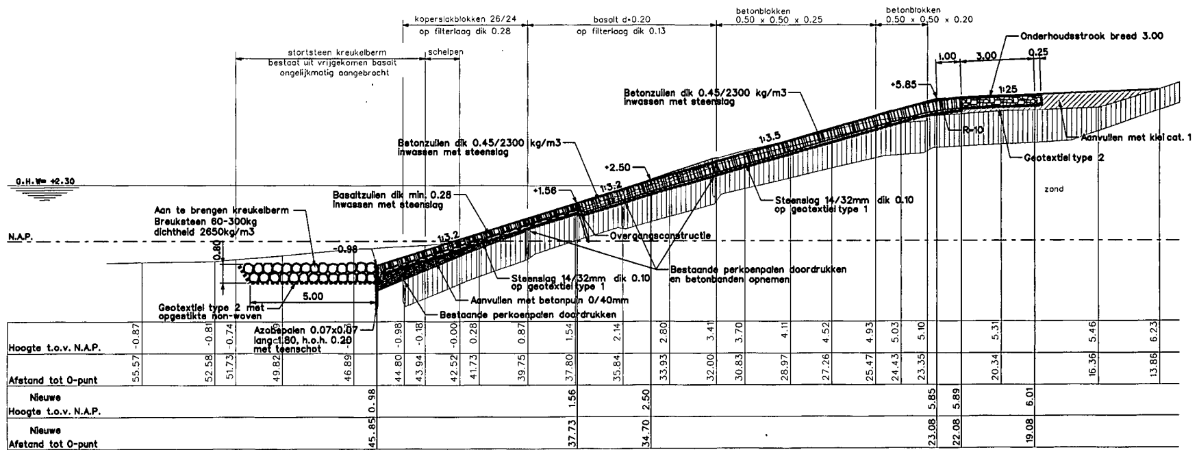
Dwarsprofiel 4 nieuw van dp90 tot dp94+85m (voor het gedeelte onder NAP +1.56 vanaf dp 90+80)
