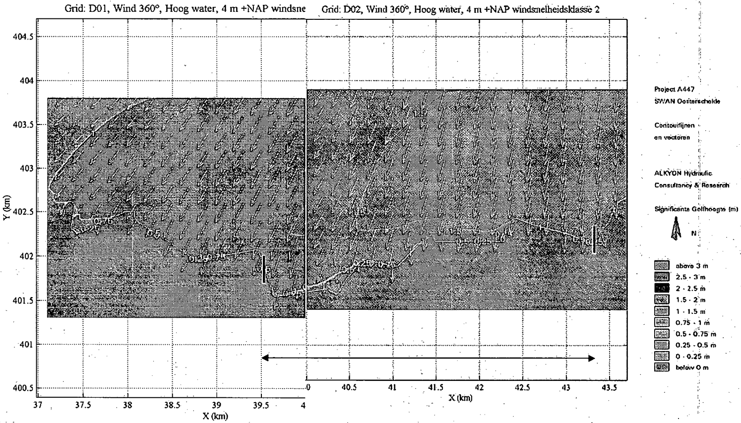
Figuur 3.2: grid D01 en D02: wind 360°, NAP +4 m
