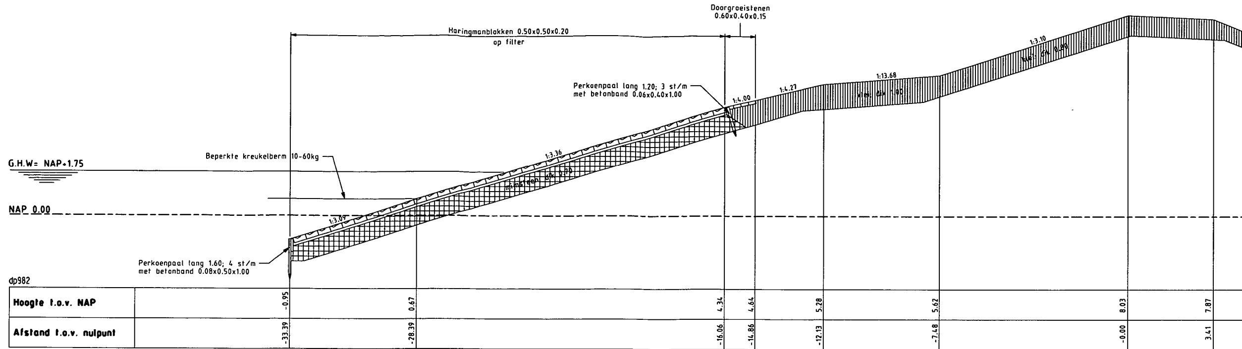
Dwarsprofiel 6 bestaand
