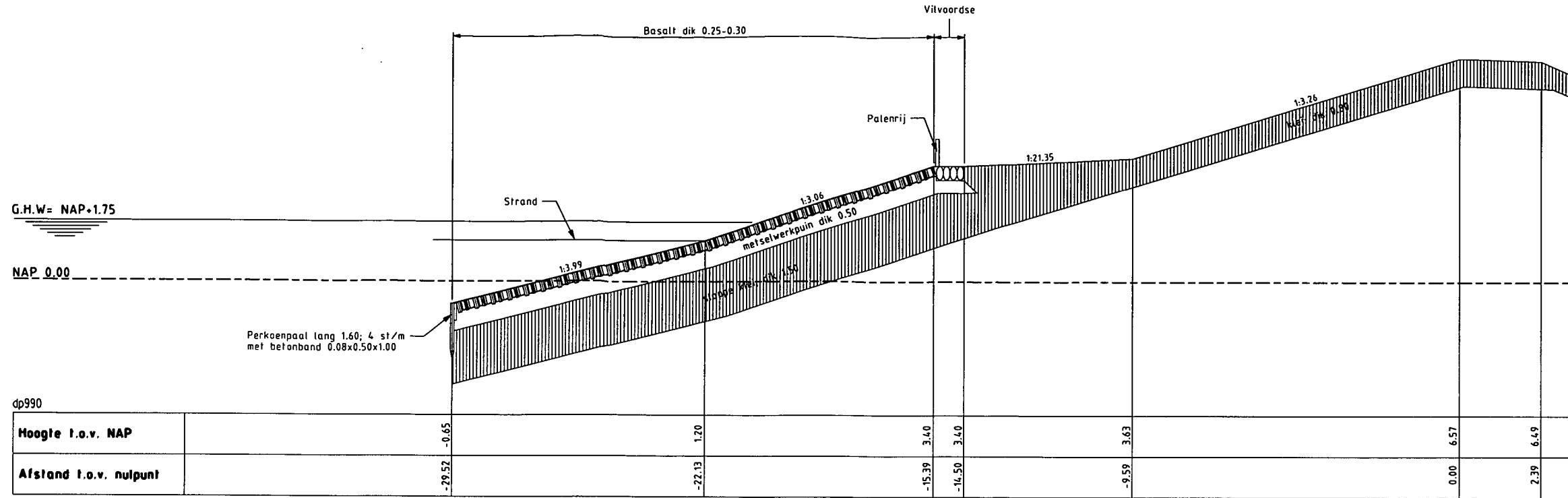
Dwarsprofiel 8 bestaand
