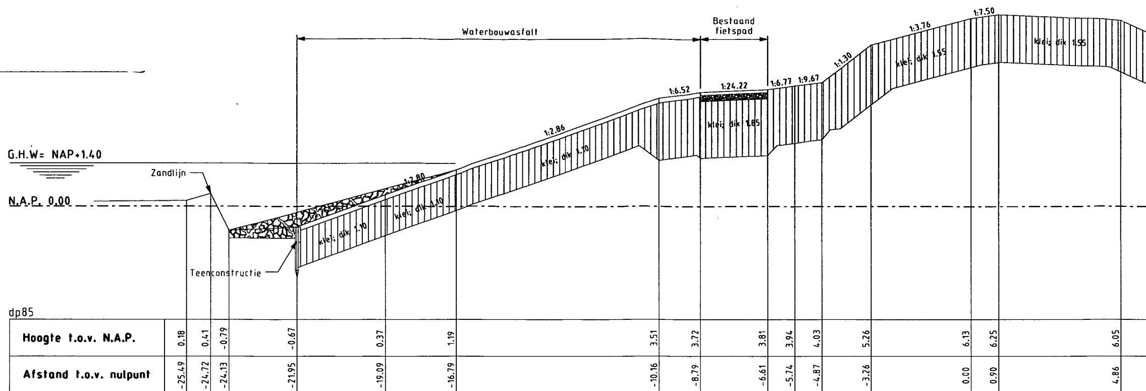
Dwarsprofiel 3 bestaand
