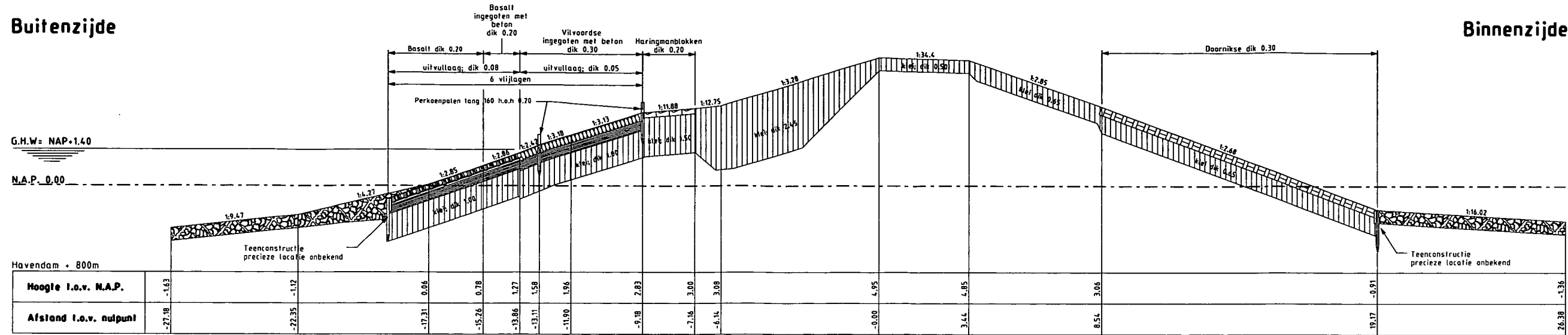
Dwarsprofiel 6 bestaand
