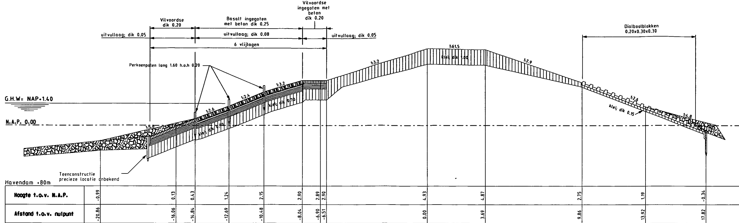
Dwarsprofiel 5 bestaand
