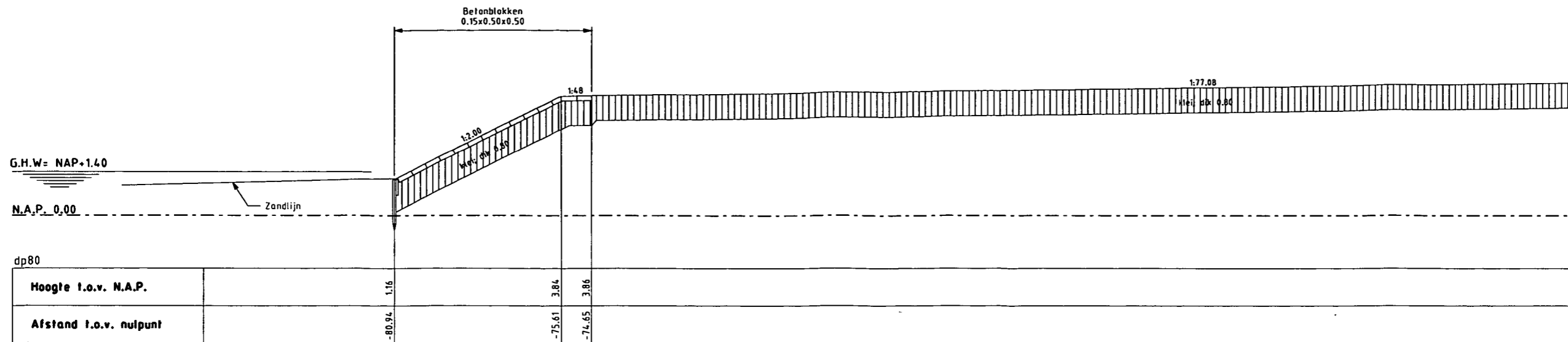
Dwarsprofiel 2 bestaand
