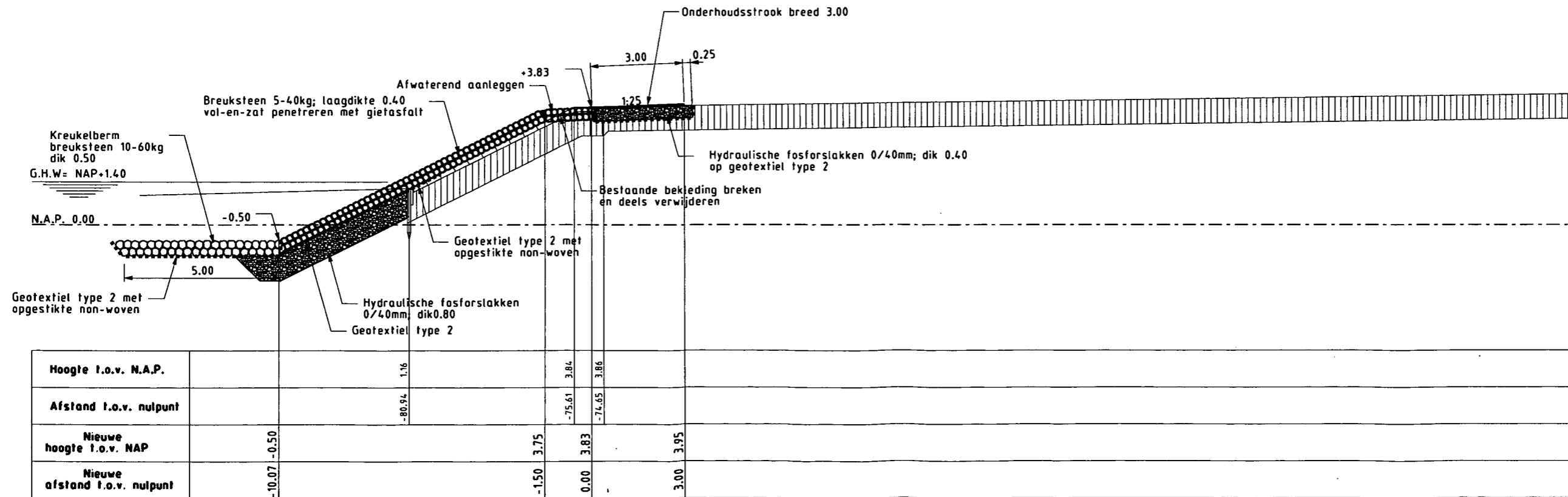
Dwarsprofiel 2 nieuw van dp79+15m tot dp81
