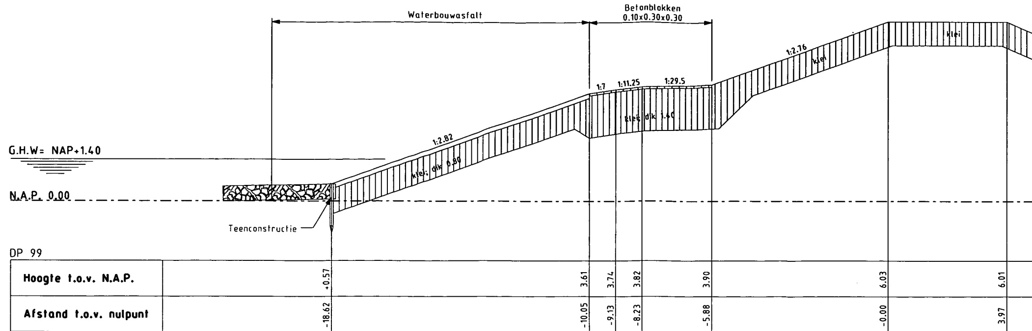
Dwarsprofiel 4 bestaand
