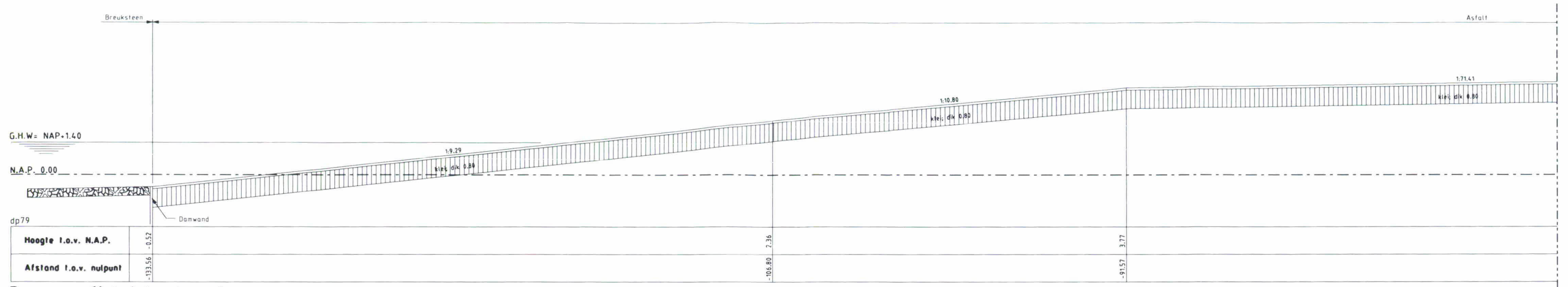
Dwarsprofiel 1 bestaand
