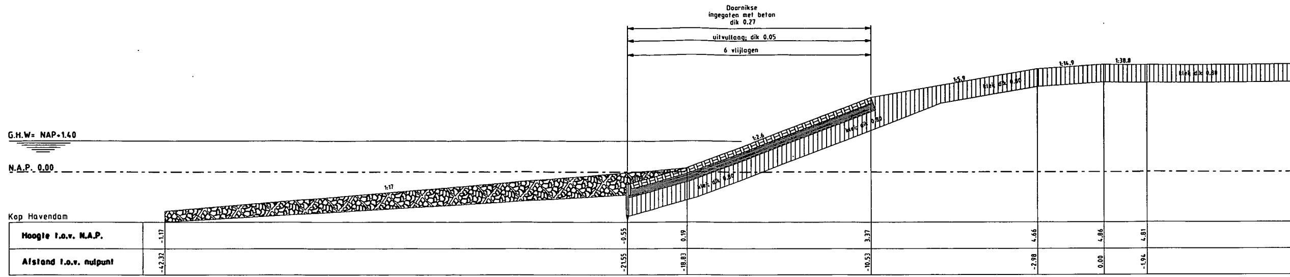
Dwarsprofiel 7 bestaand
