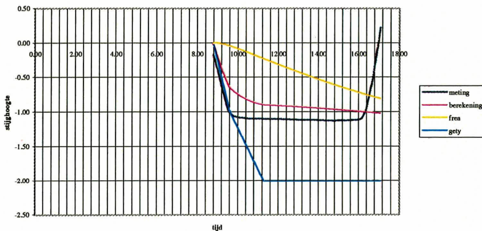
Vergelijking stijghoogtes dp8, wsm3
