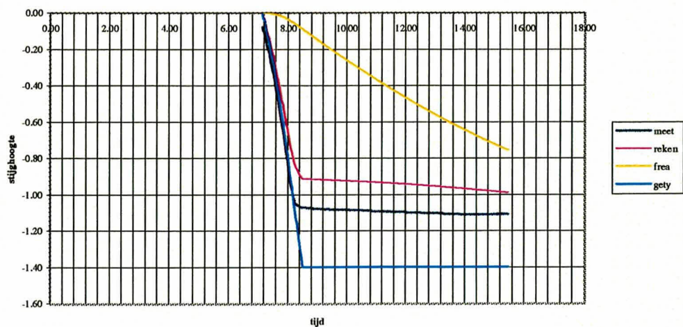
Vergelijking stijghoogtes dp6, wsm4
