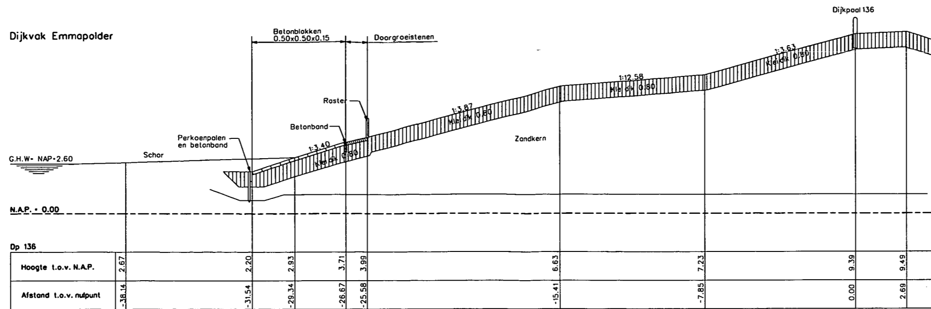
Dwarsprofiel 2 bestaand
