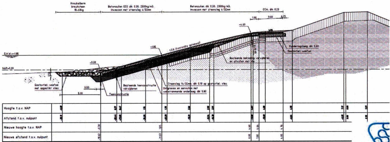
DWARSPROFIEL 1d nieuw van dp1328 tot dp1348
