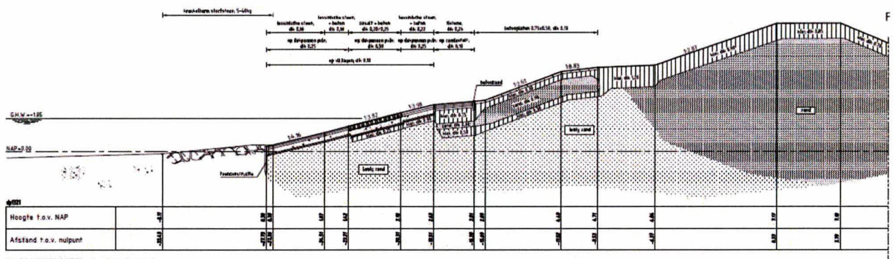
Dwarsprofiel 1a: bestaand dp 1321.
