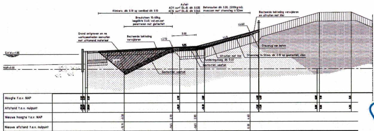
DWARSPROFIEL 1b nieuw van dp1321-23a tot dp1328-16a
