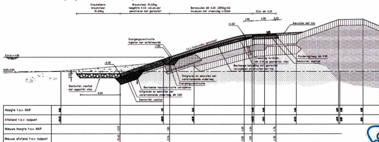
DWARSPROFIEL 3 nieuw van dp1344 tot dp1348 Dwarsprofiel 3: nieuw dp 1347.
