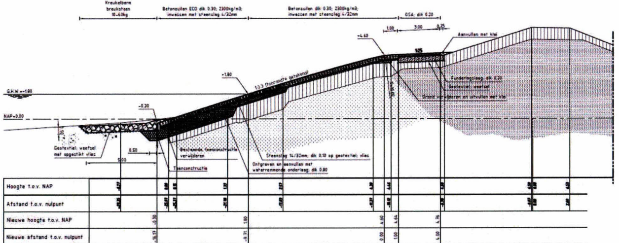
DWARSPROFIEL 2 nieuw van dp1348 tot dp1346
