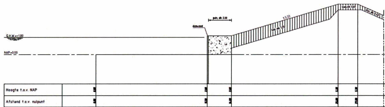
DWARSPROFIEL 4 Bestand Dwarsprofiel 4: bestand dp 1348.
