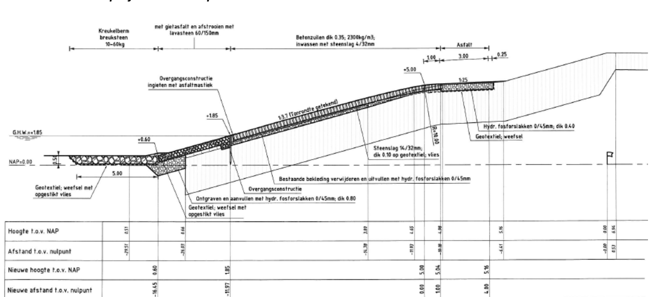
Dwarsprofiel 1: nieuw dp 1286
