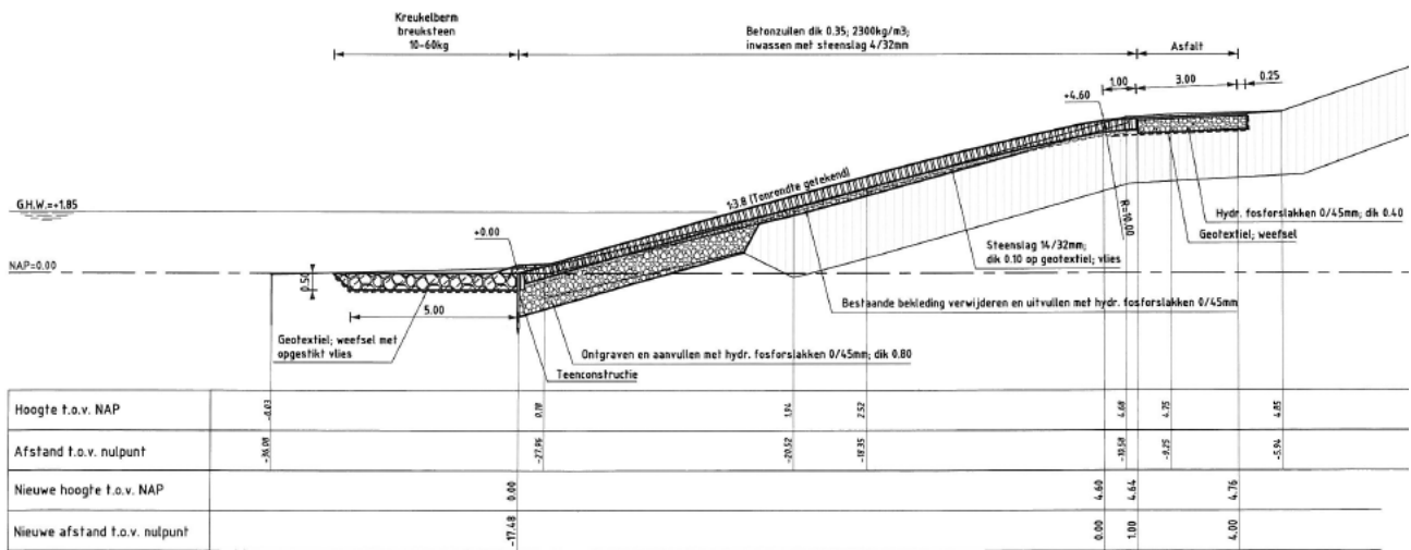
Figuur 2.2: Dwarsprofiel 1, 2 en 3 van de huidige en toekomstige steenbekleding (bron: Van der Vliet, 2011).
