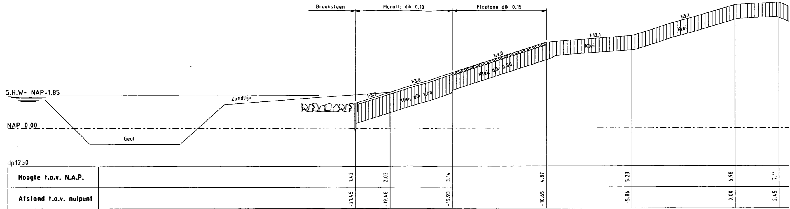
Dwarsprofiel 3 bestaand
