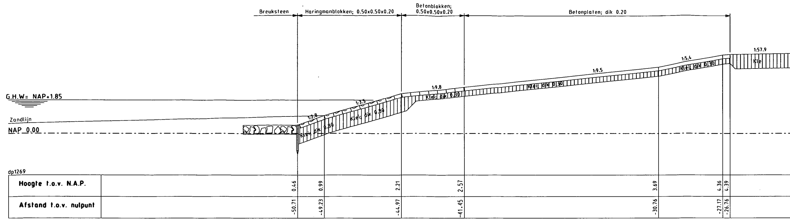
Dwarsprofiel 6 bestaand
