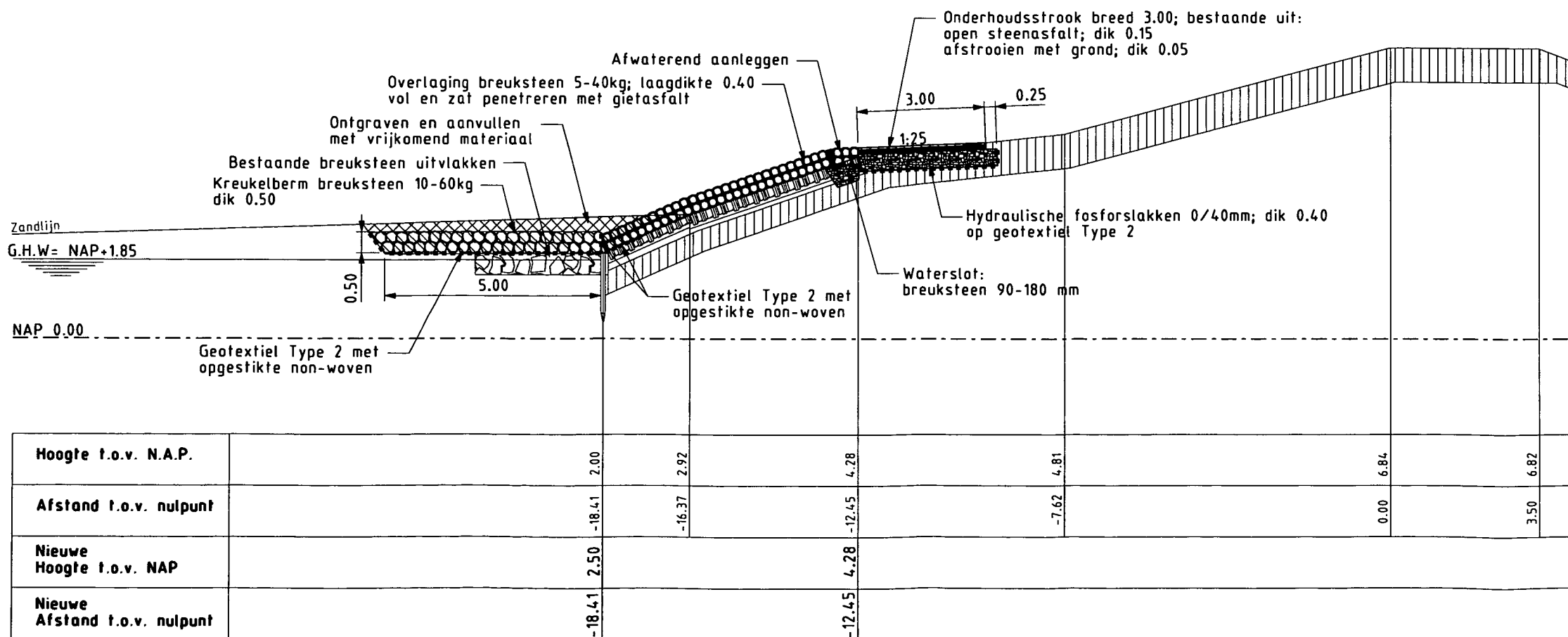
Dwarsprofiel 4 nieuw Van dp1255 tot dp1259
