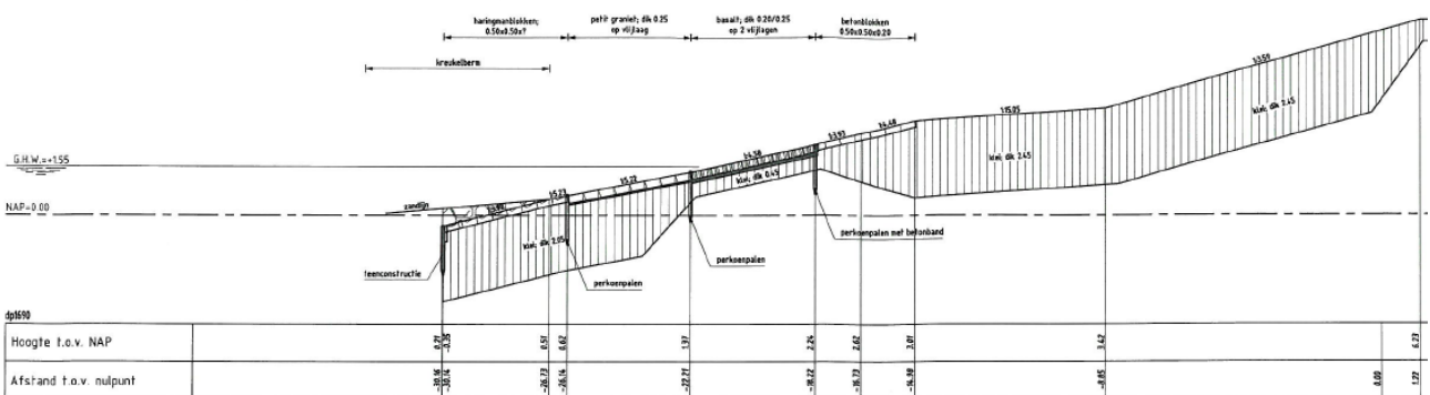
DWARSPROFIEL 2 bestaand
