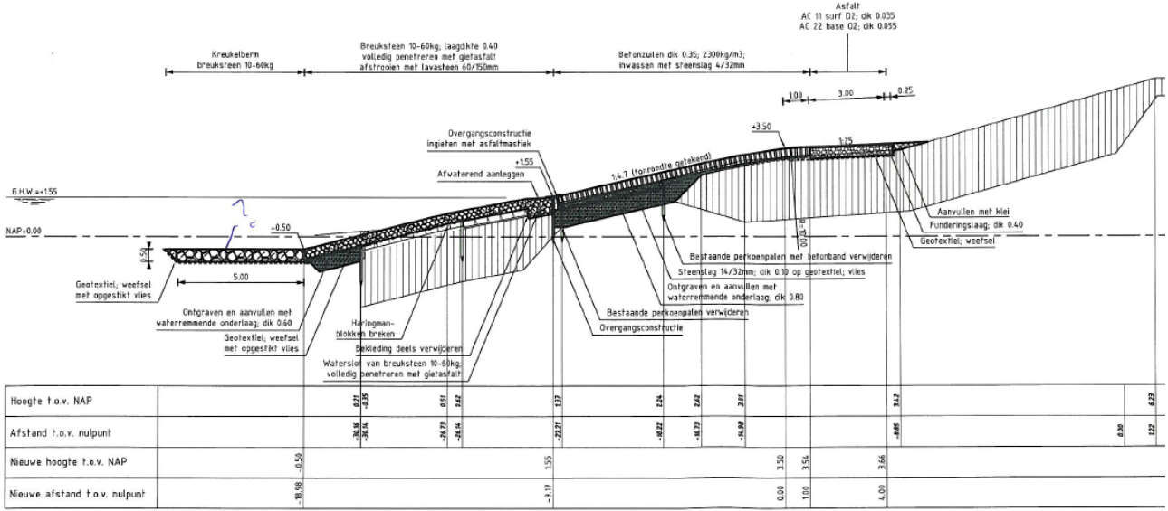
DWARSPROFIEL 2a nieuw van dp1685 tot dp1699
