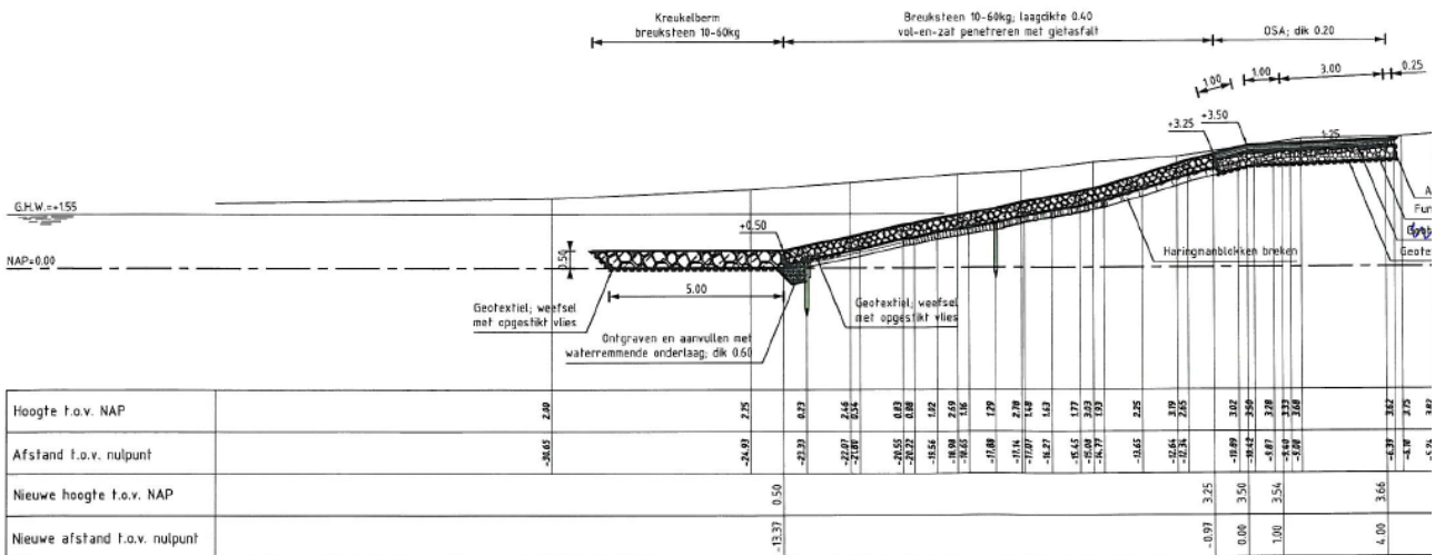
DWARSPROFIEL 3 nieuw van dp1699 tot dp1702-50m
