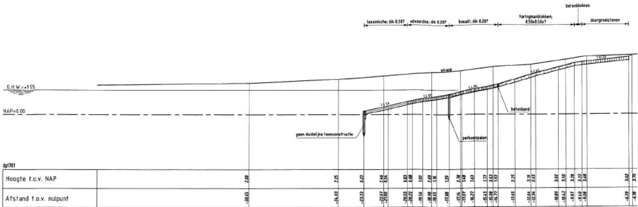
DWARSPROFIEL 3 bestaand
