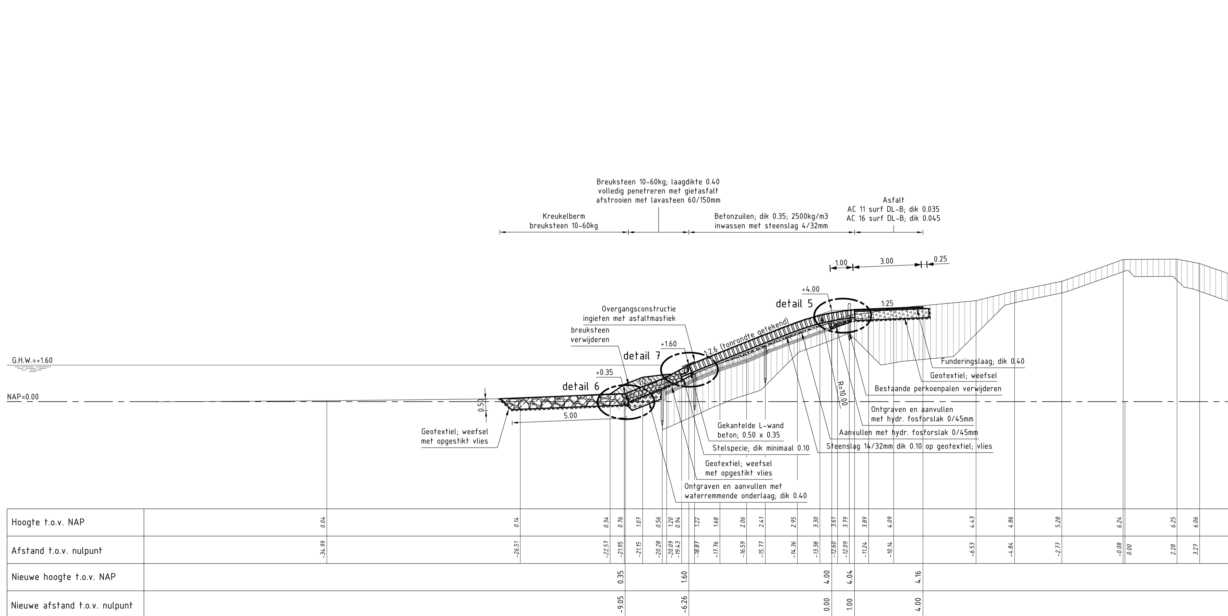
DWARSPROFIEL 3 nieuw van dp813+38m tot dp816+45m
