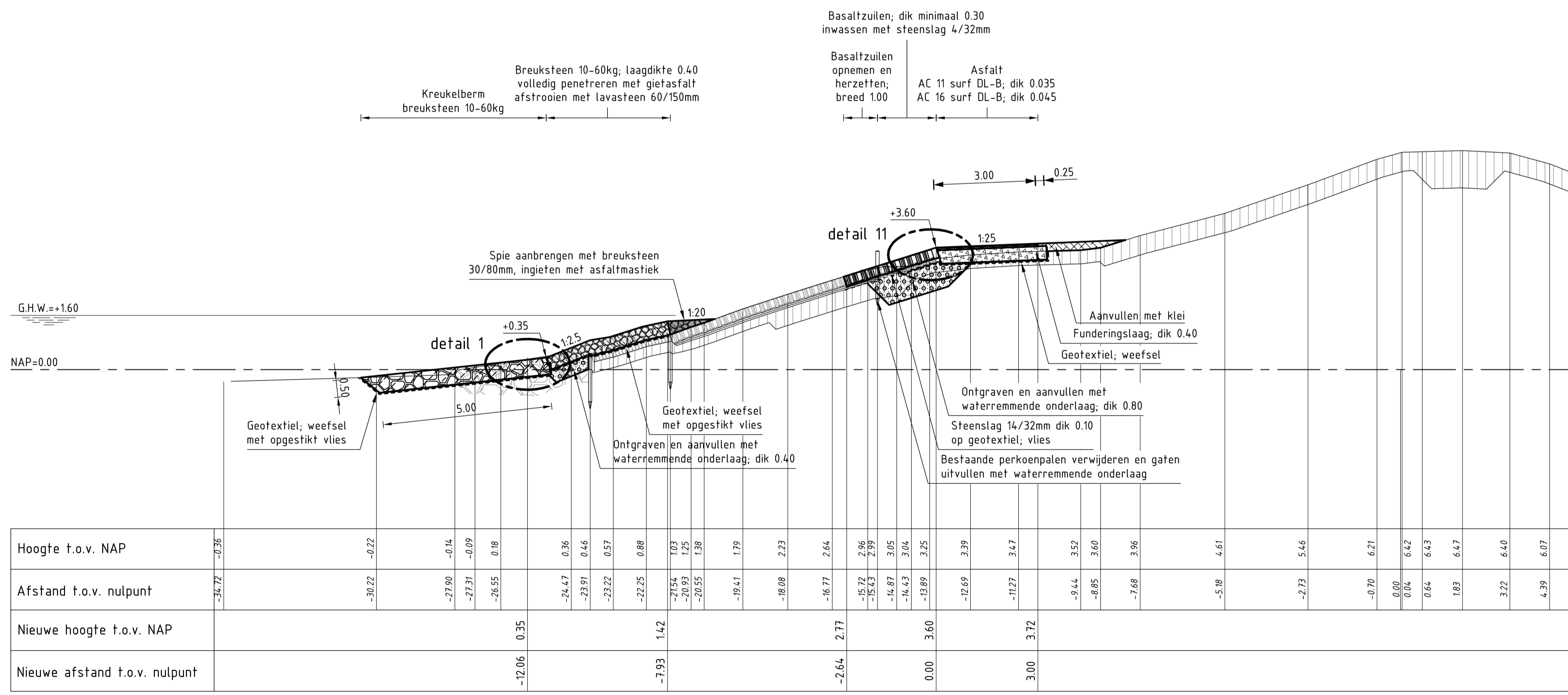
DWARSPROFIEL 6 nieuw schaal 1:100 van dp820+70m tot dp836 geen overlaging, wel kreukelberm aanbrengen van: - dp820+70m t/m dp822+78m - dp824+36m t/m dp826+5m - dp828+40m t/m dp831 - dp834+66m t/m dp836
