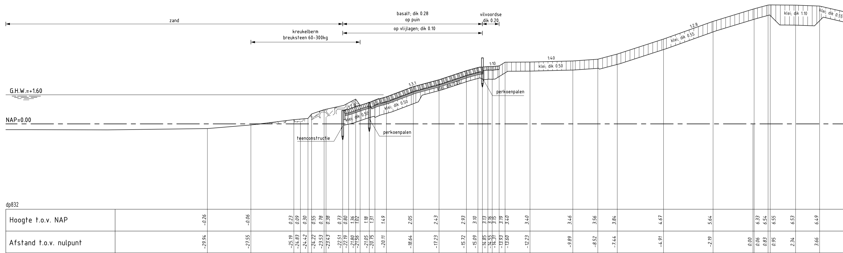
DWARSPROFIEL 7 bestaand schaal 1:100
