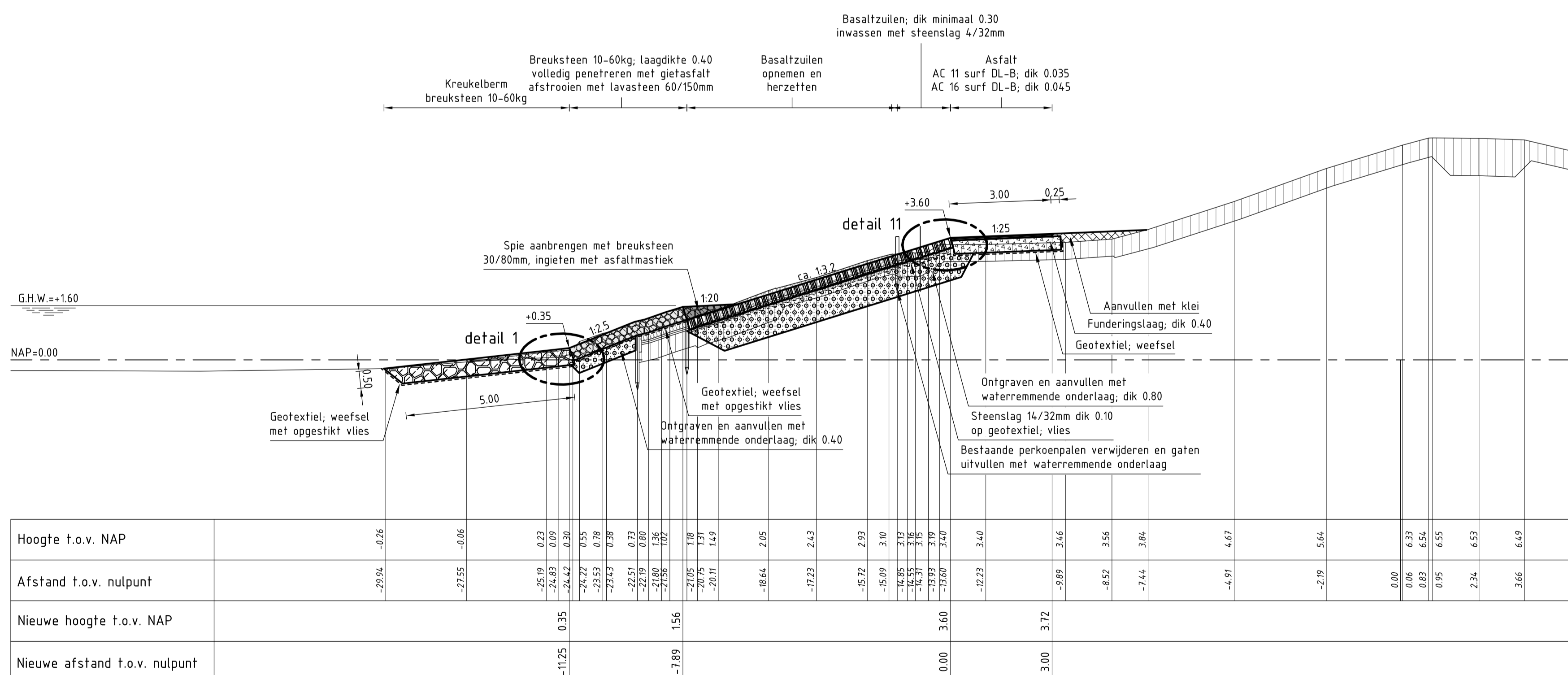
DWARSPROFIEL 7 nieuw van dp831 tot dp833+35m schaal 1:100
