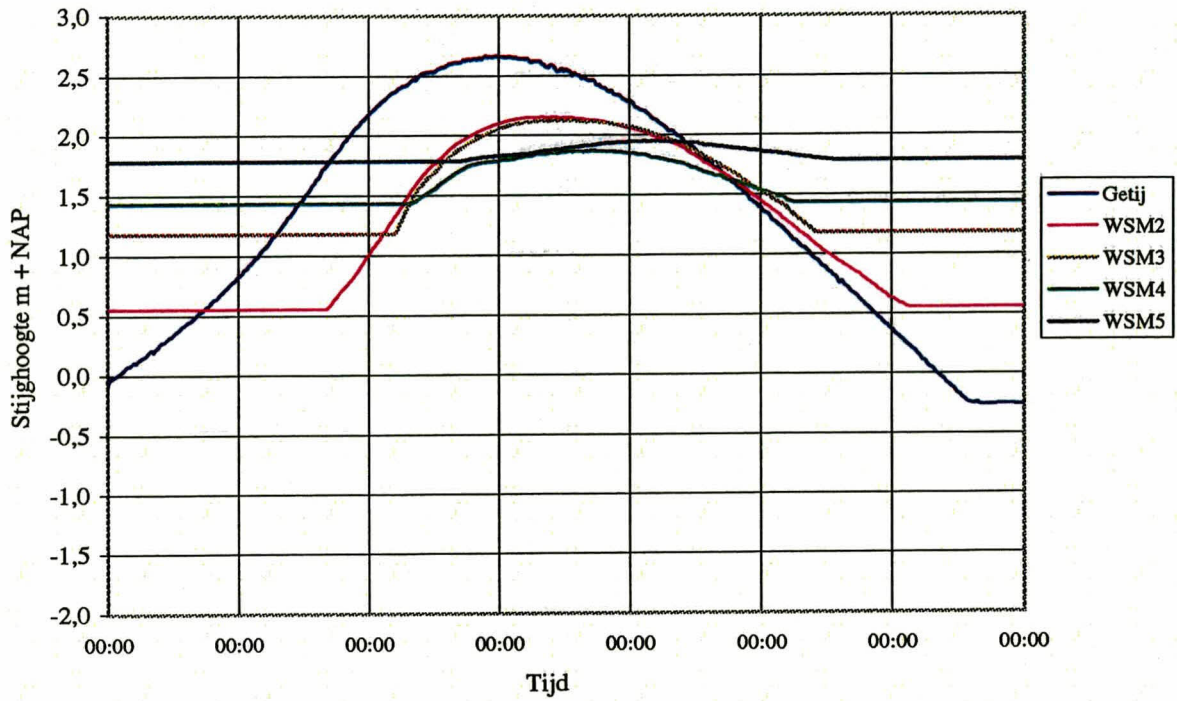
Stijghoogteverloop Inkelenvolder, raai G1
