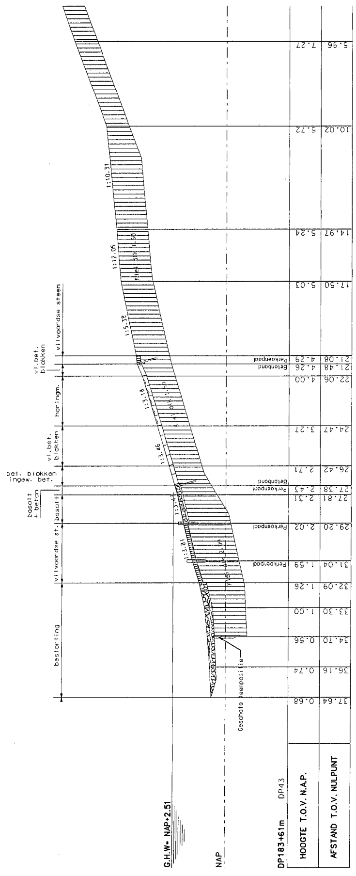
Dwarsprofiel 11 bestaand
