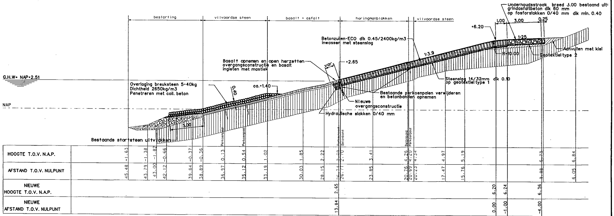
Dwarsprofiel 10 nieuw van dp175 tot 180+80m
