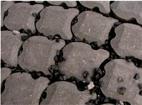
Goed aangevulde betonzuilen
