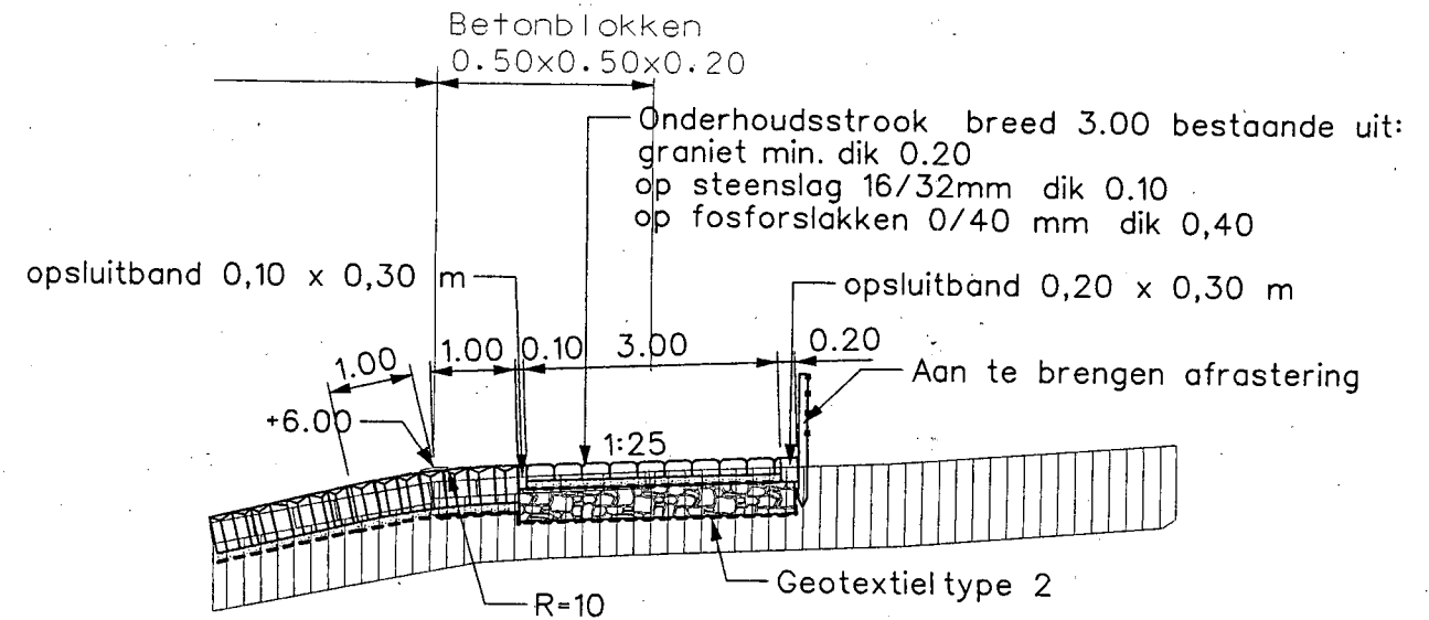
Onderhoudstrook alternatief 2 schaal 1:100
