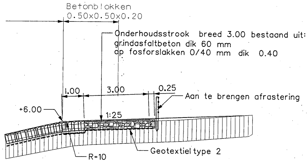
Onderhoudstrook alternatief 1 schaal 1:100
