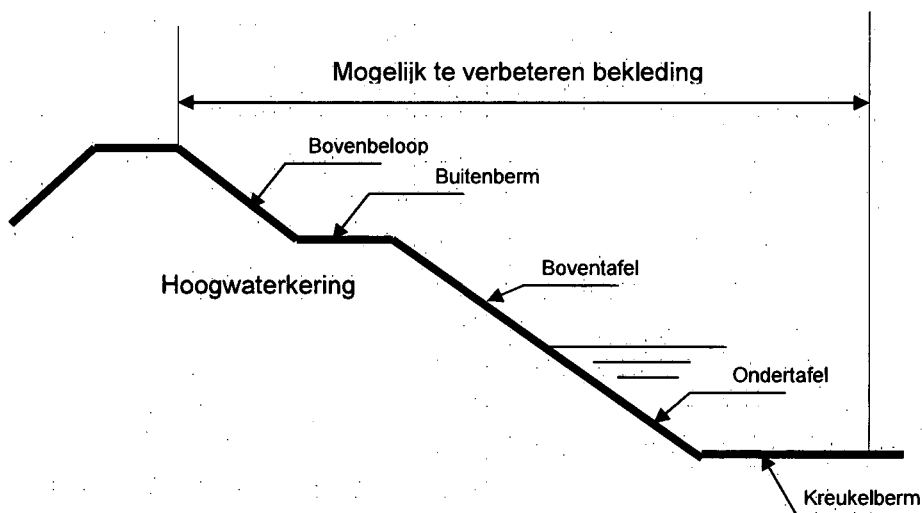
Figuur 2.1. Schematische weergave van het dijklichaam
