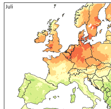
Figuur 7.4 Gesimuleerde afwijking van het neerslagtekort in het future weather-experiment met (a) 2018 in het huidige klimaat, en (b) 2018 in een 2°C opgewarmd klimaat. Afwijking ten opzichte van de klimatologie 1991-2020, kaartjes laten de waarde op de laatste dag van de maand zien.
