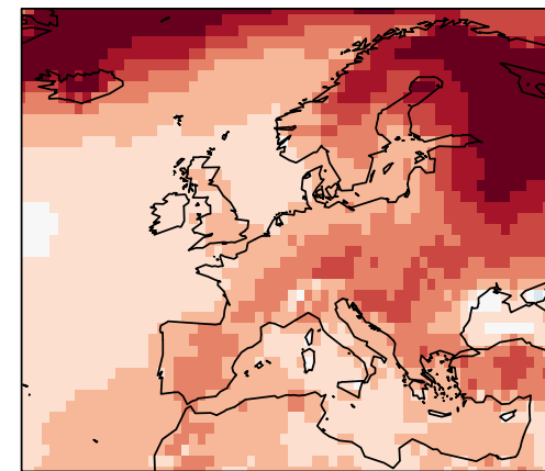
Trendbijdrage: mondiale opwarming (winter)
