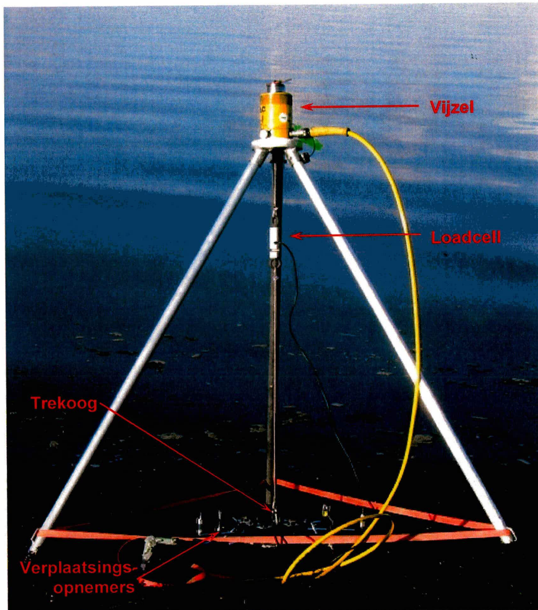
Fig 2.1 overzicht meetopstelling en trekstoel
