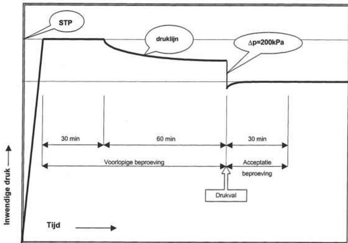
Figuur 14 Voorbeeld van de acceptatiebeproeving van leidingen met visco-elastisch gedrag.
