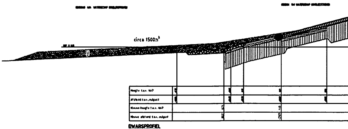
Afbeelding 2: Dwarsprofiel van het nieuwe strand langs de Stormesandepolder.
