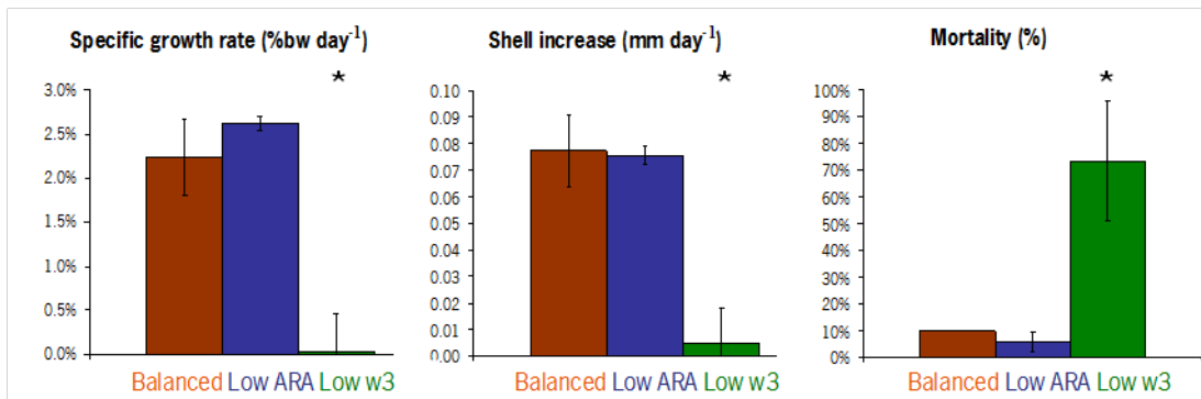
Fig. 4.3.1a Groeisnelheid en sterfte van kokkels aan het einde van het eerste voer experiment gevoerd met 3 diëten: Balanced = EPA, DHA en ARA; Low ARA = EPA en DHA en Low w3 = geen EPA, DHA of ARA). Gemiddelde met sd (n=3).
