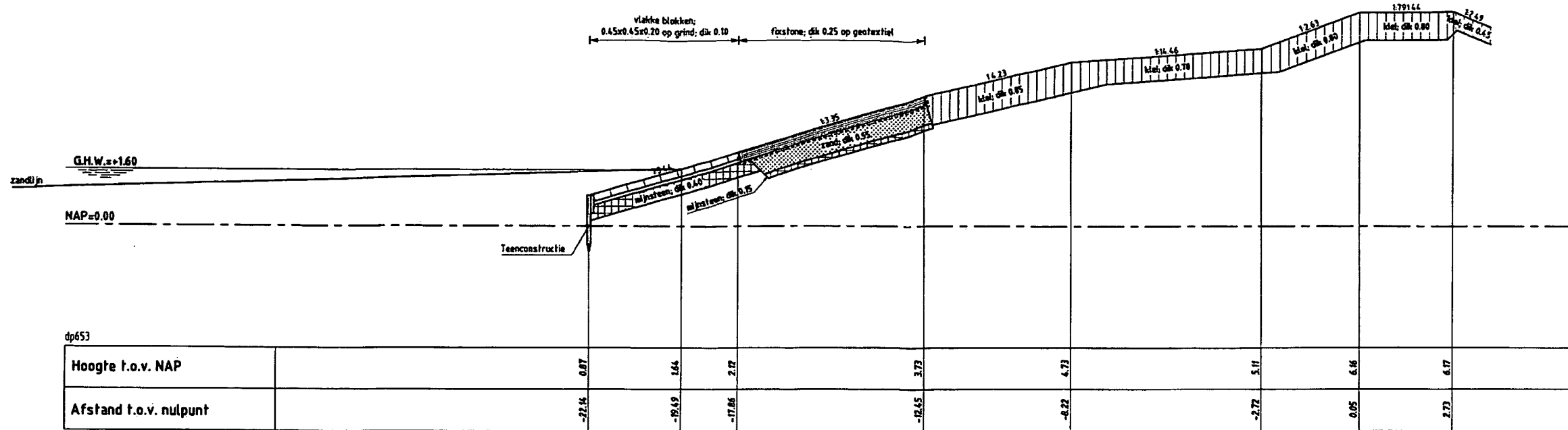
DWARSPROFIEL 4 bestand
