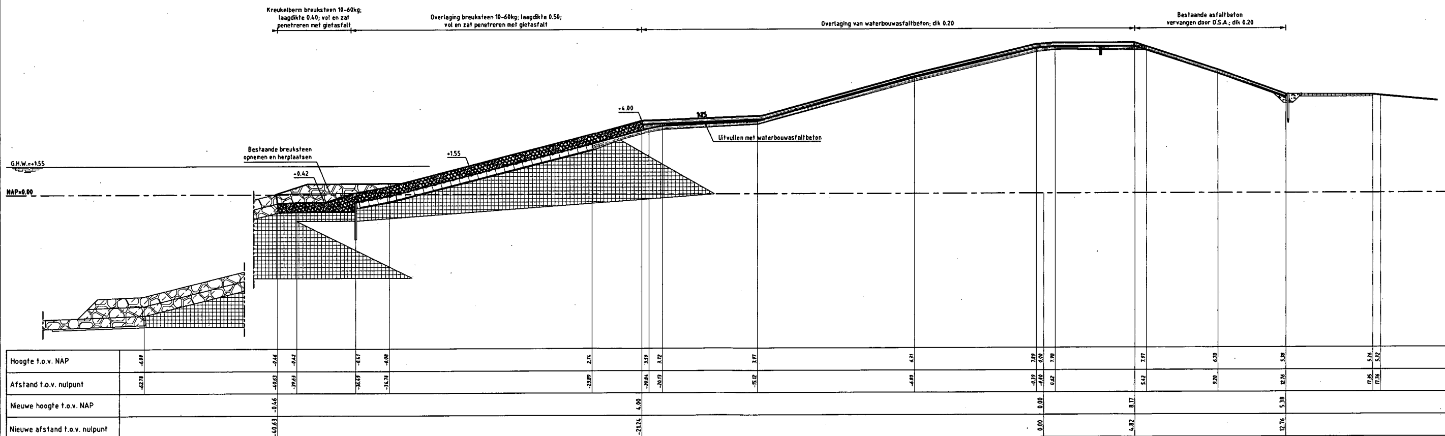
DWARSPROFIEL 2 nieuw Van dpl=58m tot dpl=80m
