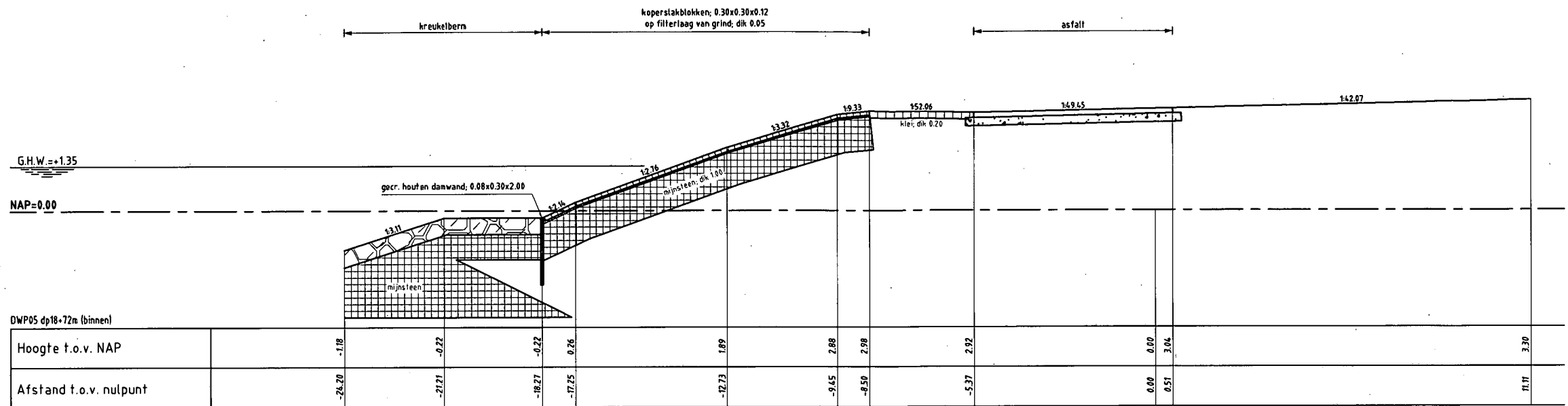
DWARSPROFIEL 5 bestaand
