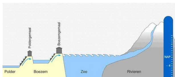
Stelsel van polder, boezem en gemalen
