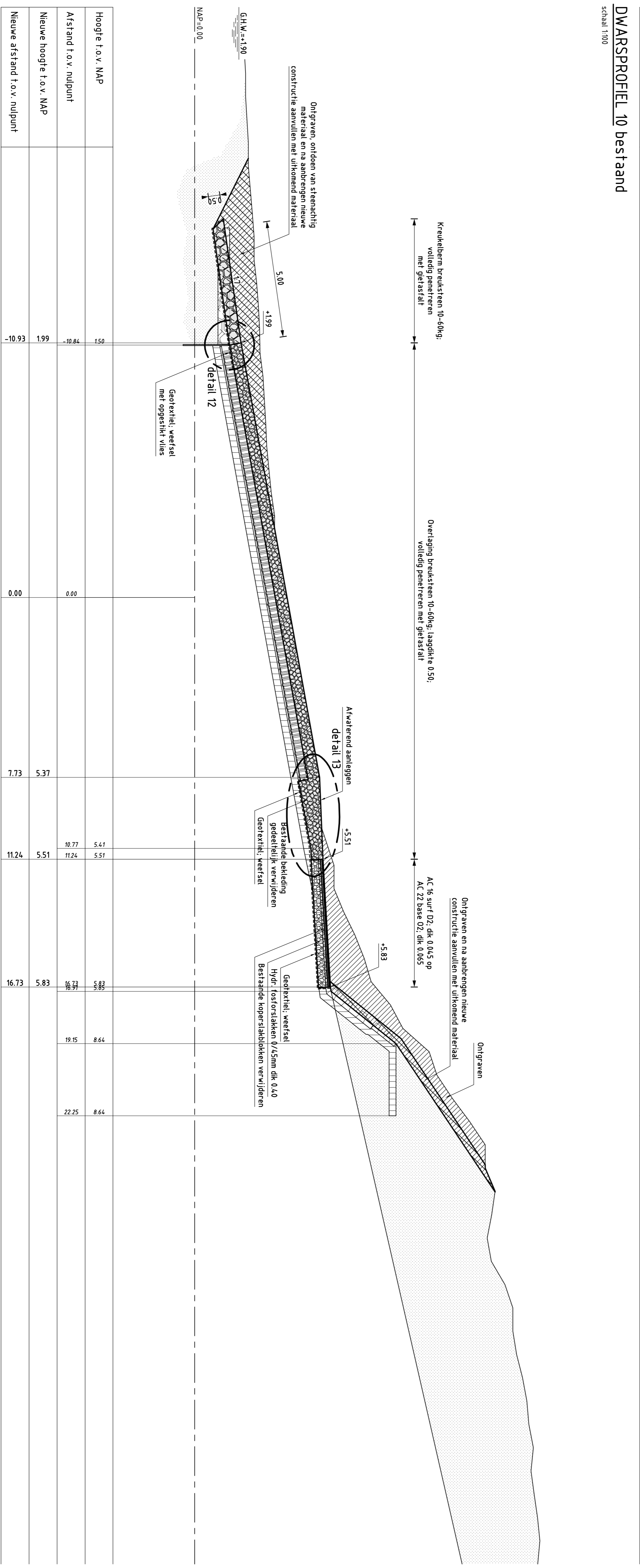
DWARSPROFIEL 10 nieuw van dp224 tot dp224-50m schaal 1:100
