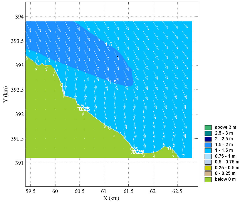
Grid: D10, Wind 360°, Hoog water, 4 m +NAP windsnelheidsklasse 2
