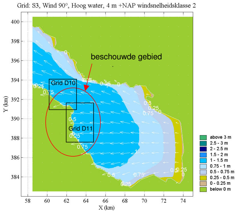
Figuur 2.1 t/m 2.3: SWAN resultaten (groot rooster)
