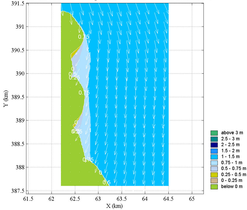
Grid: D11, Wind 360°, Hoog water, 4 m +NAP windsnelheidsklasse 2
