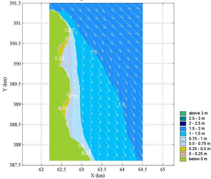
Grid: D11, Wind 300°, Hoog water, 4 m +NAP windsnelheidsklasse 2
