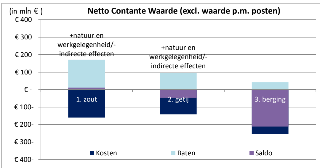
Figuur 15: NCW van bouwstenen als de waterkwaliteit in het Volkerak-Zoommeer autonoom wel verbeterd, alle baten starten in 2020
