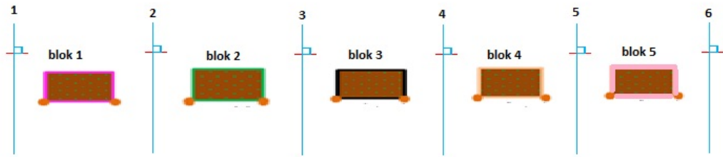
Figuur 32. Plaats van de erosiepinen bij Zuidgors, ieder blok vertegenwoordigt één replica met 8 vierkante meters. Totaal 5 replica's, met aanduiding (bruine hoekpunten) voor de meetpunten voor de dGPS.
