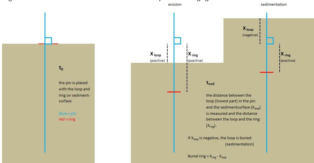
Figuur 31. Meetmethode met erosiepinnen bij Zuidgors.
