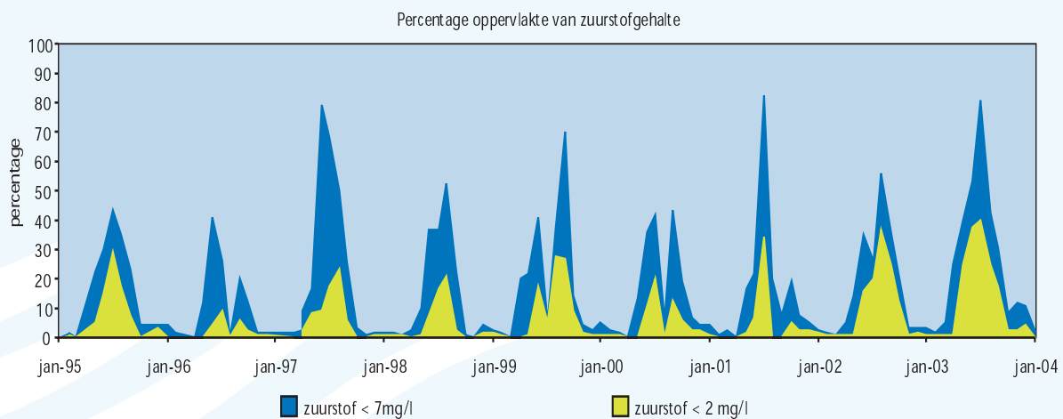
Figuur 3.5 Percentage oppervlakte zuurstofarme delen.
