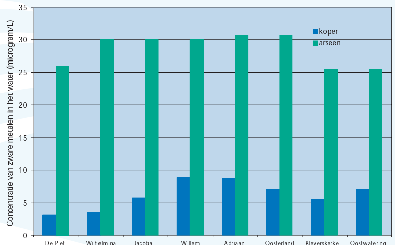
Figuur 3.15 Jaargemiddelde gehalten van koper en arseen in polderwater bij gemalen rond het Veerse Meer in 1999.
