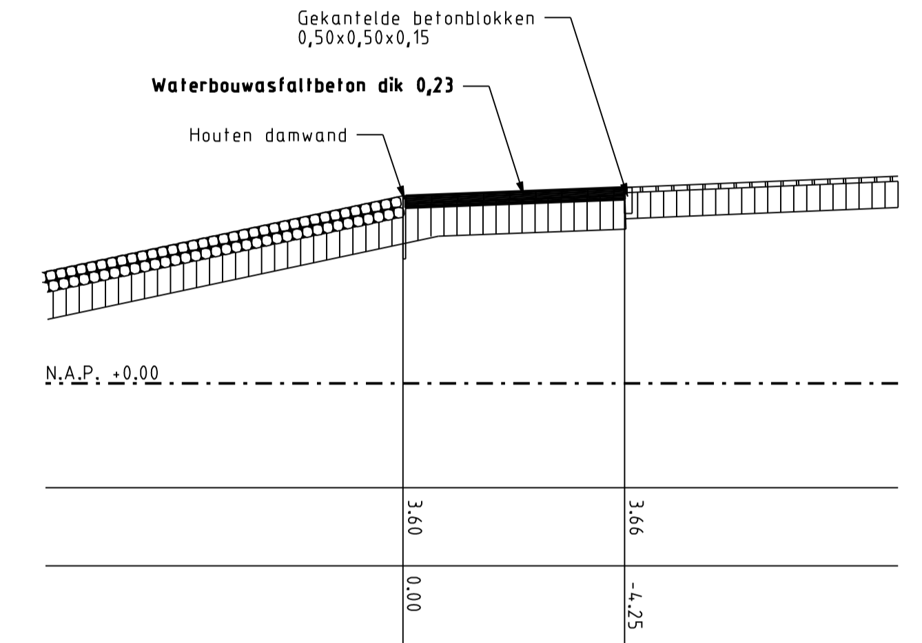
Dwarsprofiel 2 nieuw Schaal 1:100
