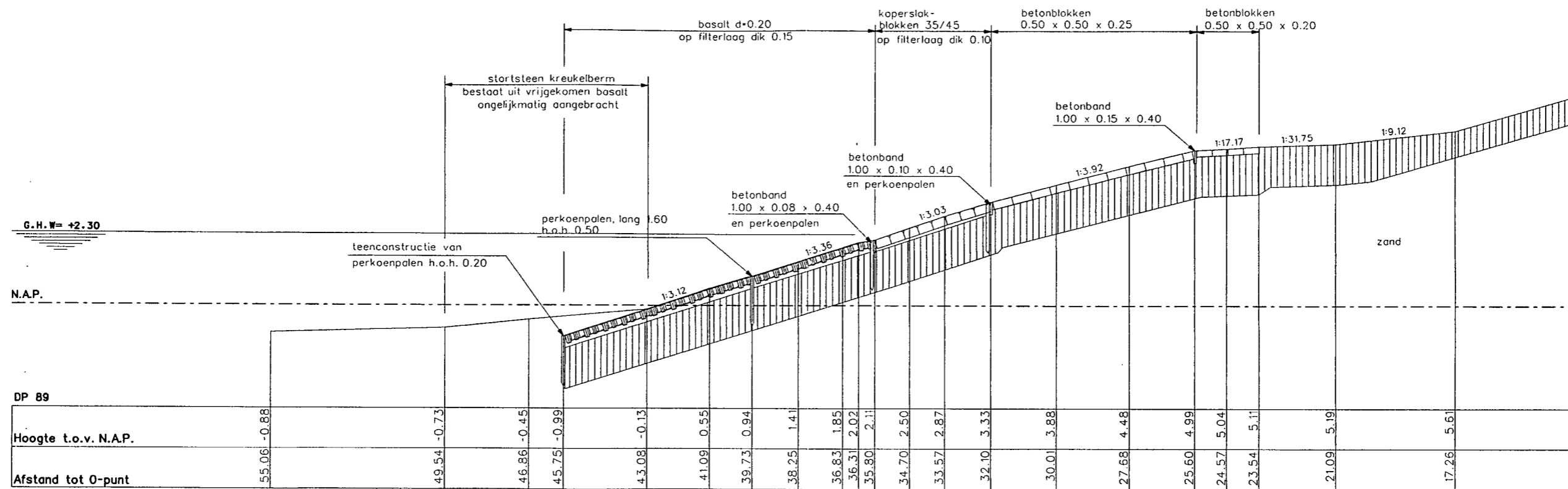
Dwarsprofiel 3 bestand
