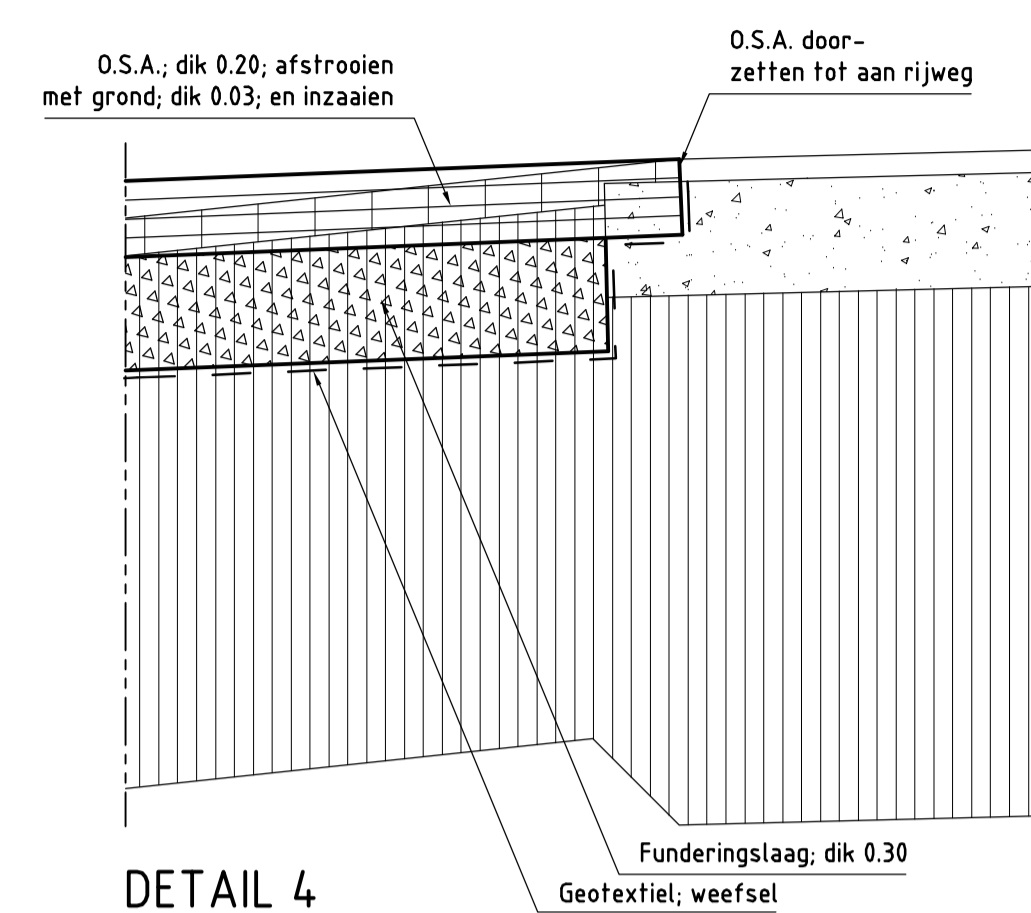
DETAIL 4 schaal 1:20
