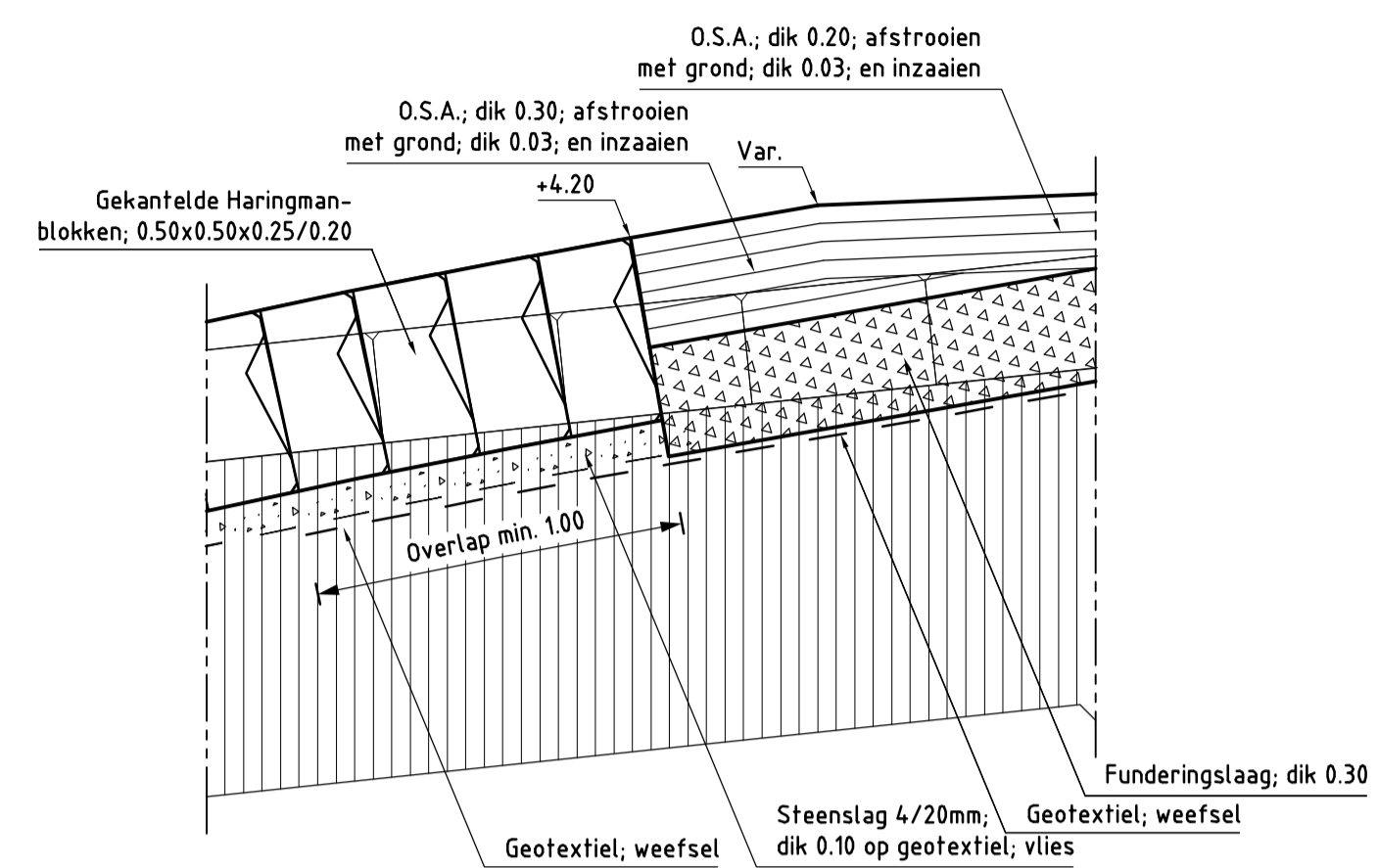
DETAIL 3 schaal 1:20
