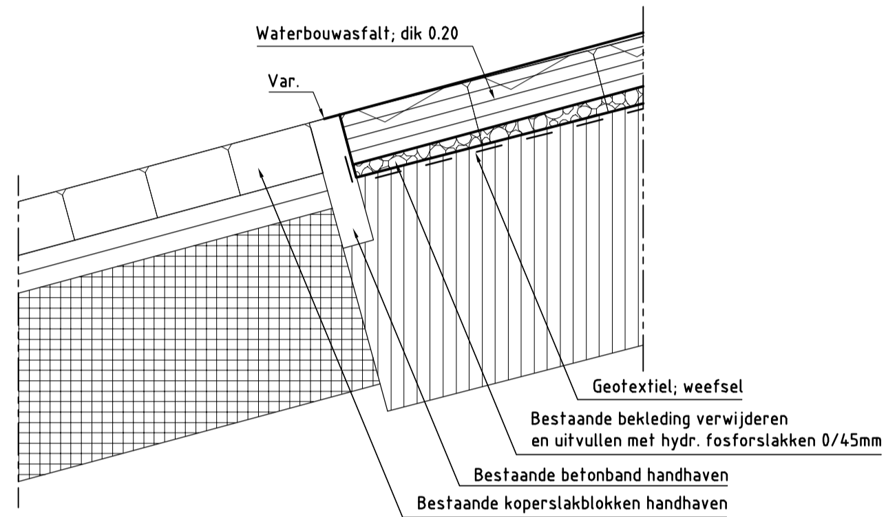
DETAIL 1 schaal 1:20
