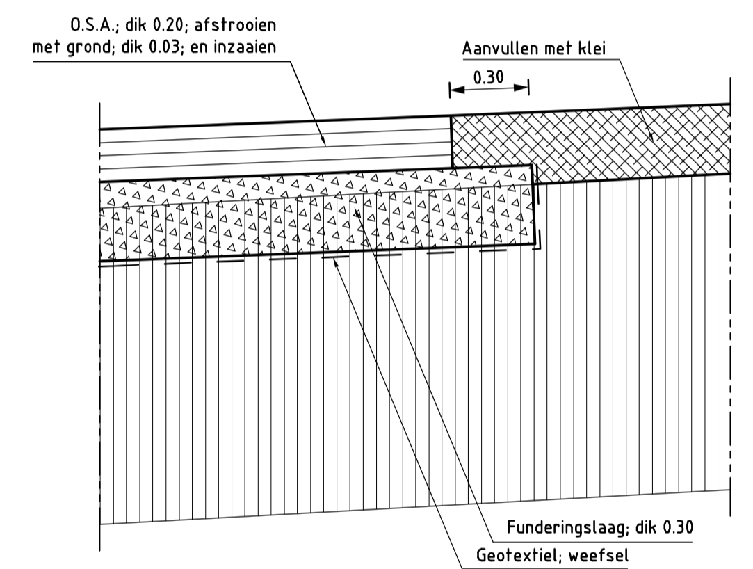
DETAIL 5 schaal 1:20
