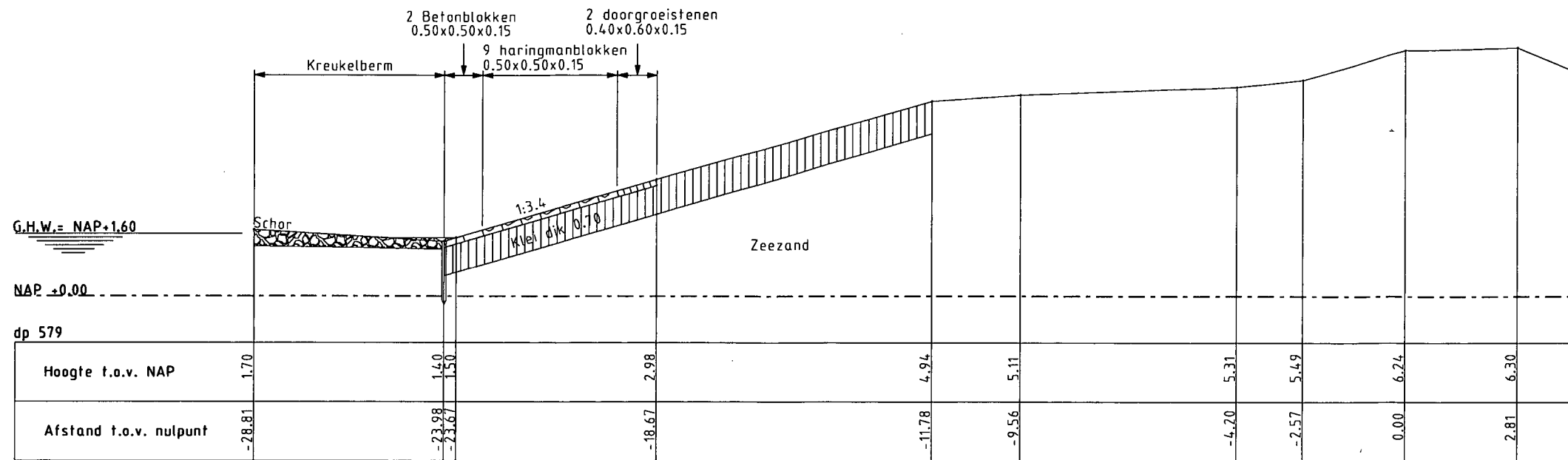
Dwarsprofiel 6 bestaand
