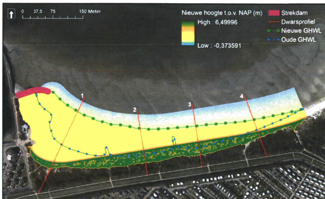
Afbeelding 6: Hoogte en overzicht van dwarsprofielen bij suppletie.
