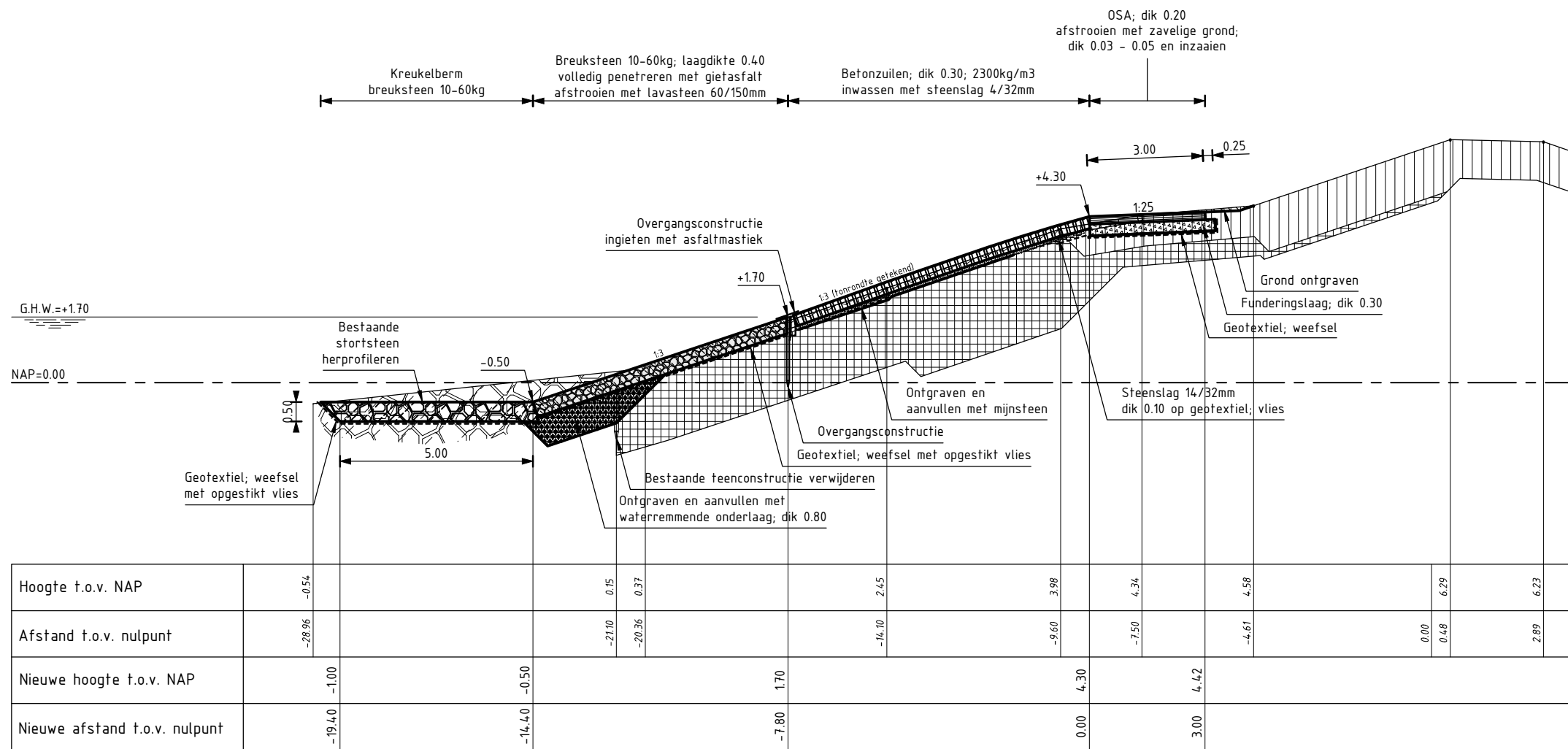
DWARSPROFIEL 2 nieuw van dp711+50m tot dp714+49m
