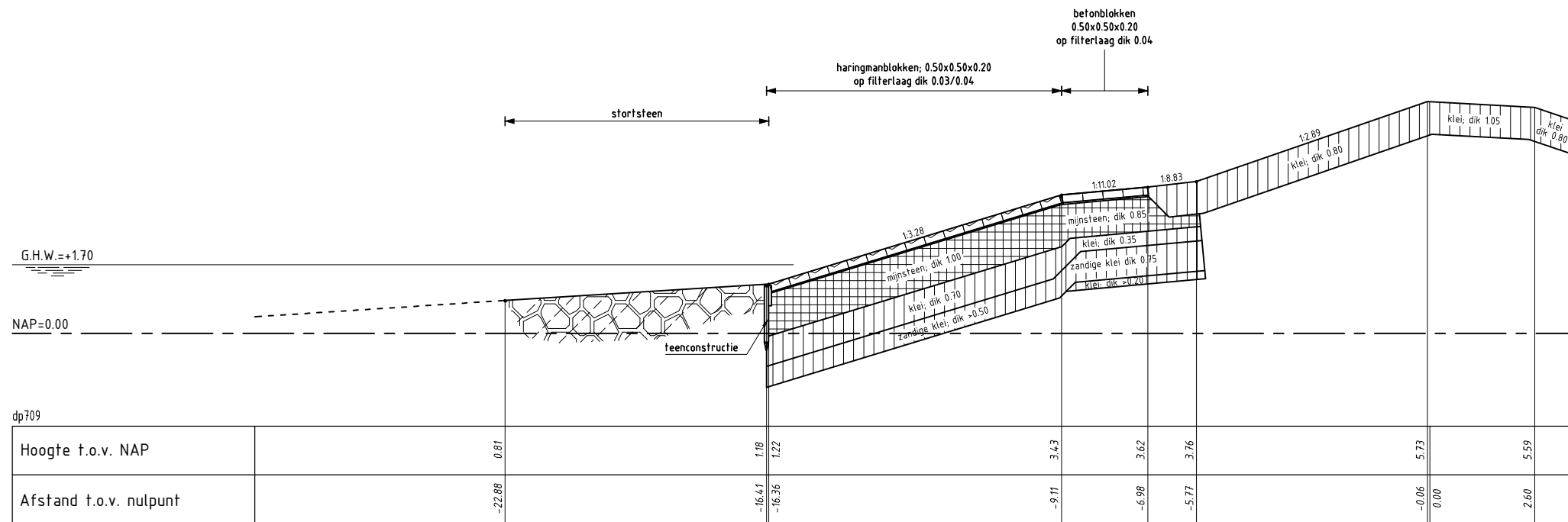
DWARSPROFIEL 1 bestand
