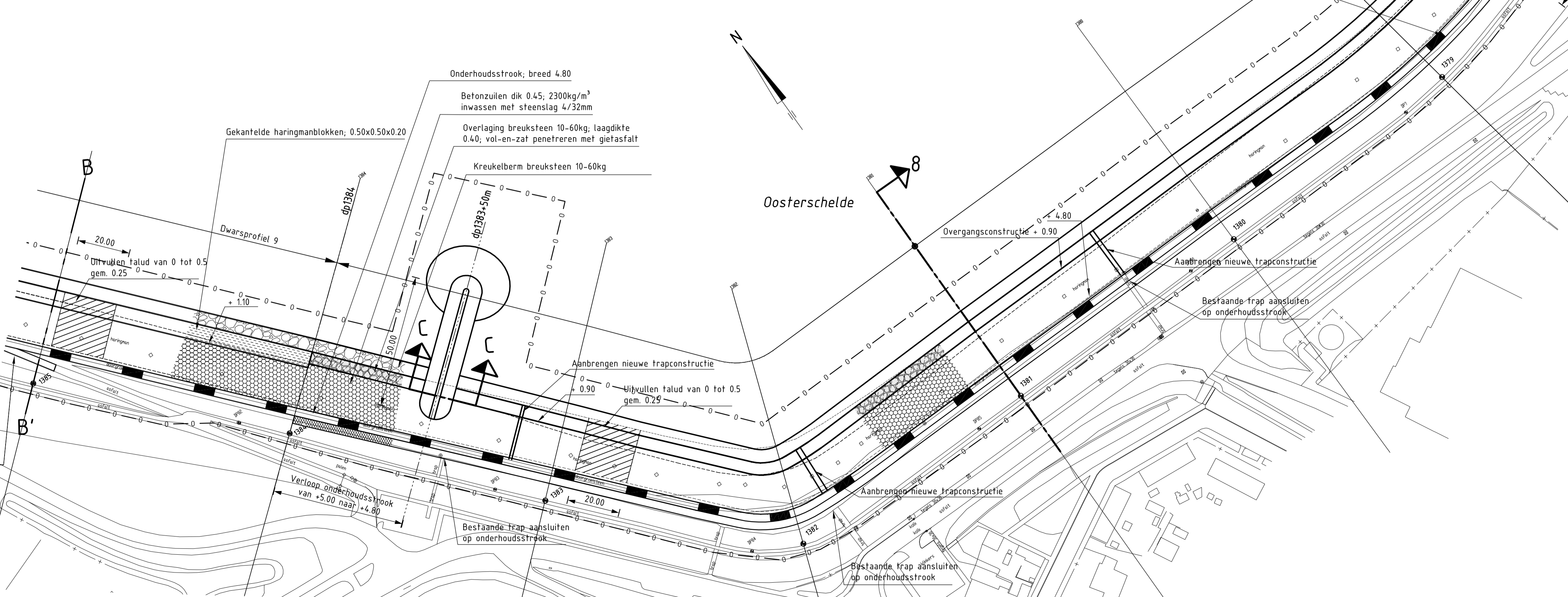
SITUATIE nieuw schaal 1:1000
