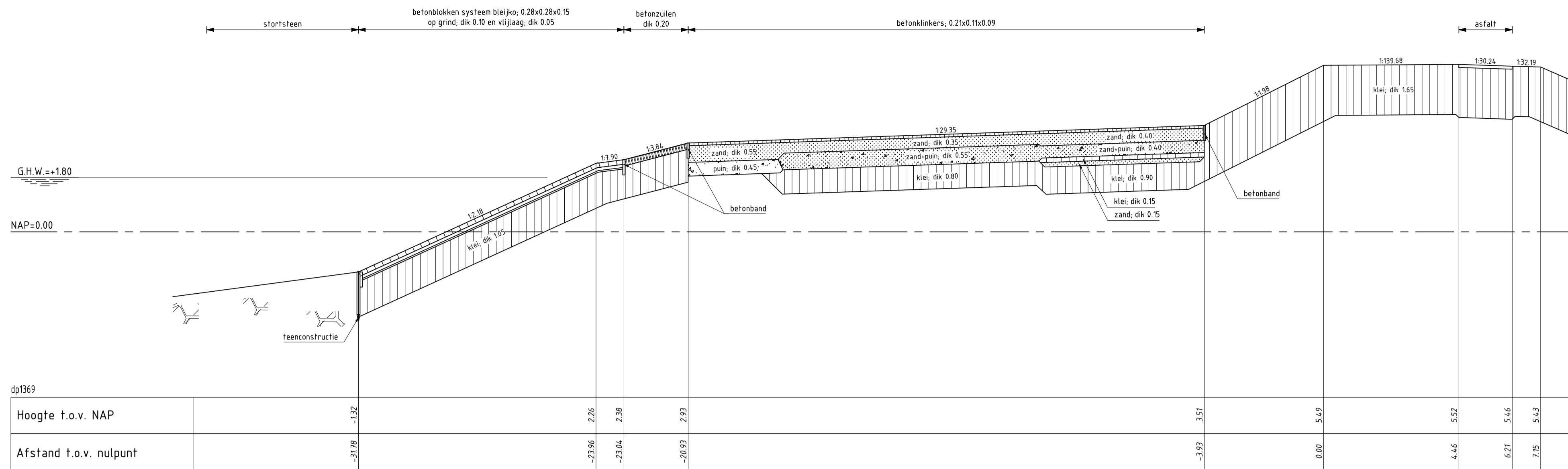
DWARSPROFIEL 3 bestaand
