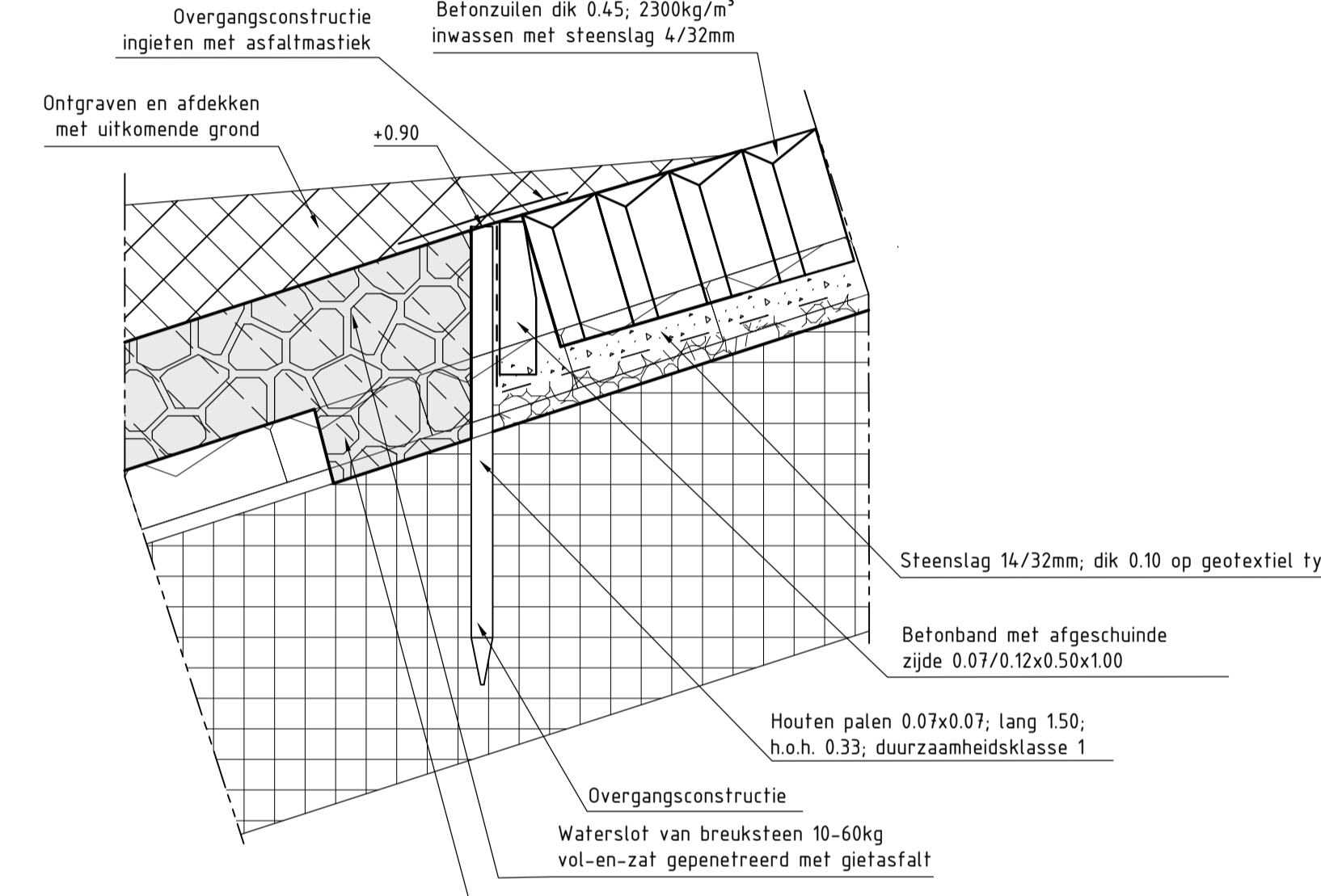
DETAIL 7 schaal 1:20
