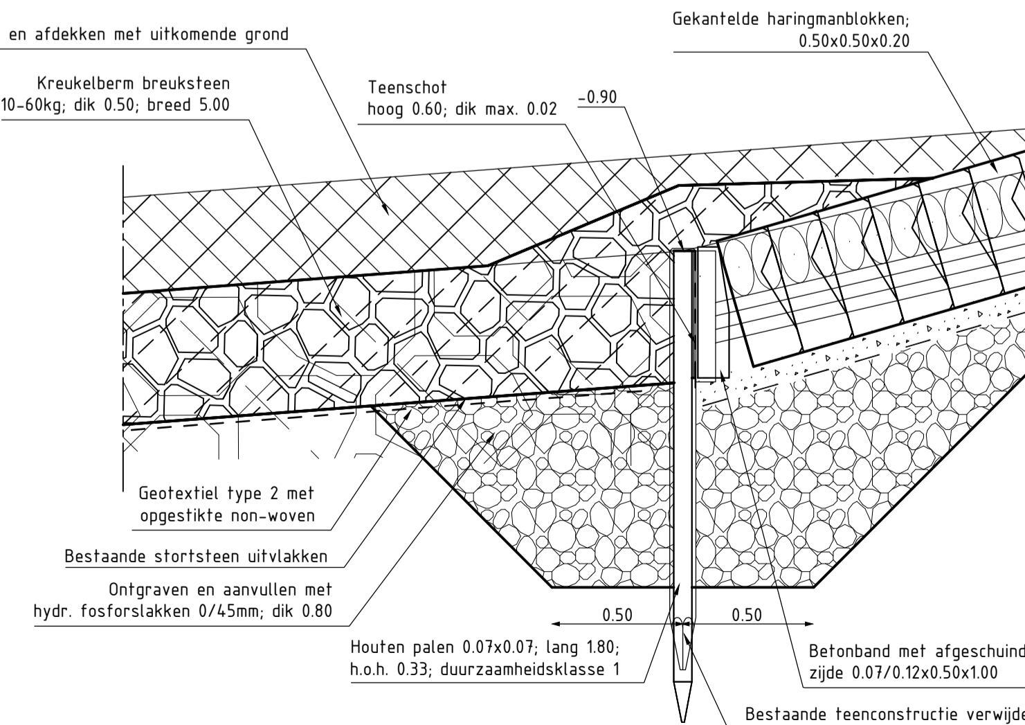
DETAIL 8 schaal 1:20
