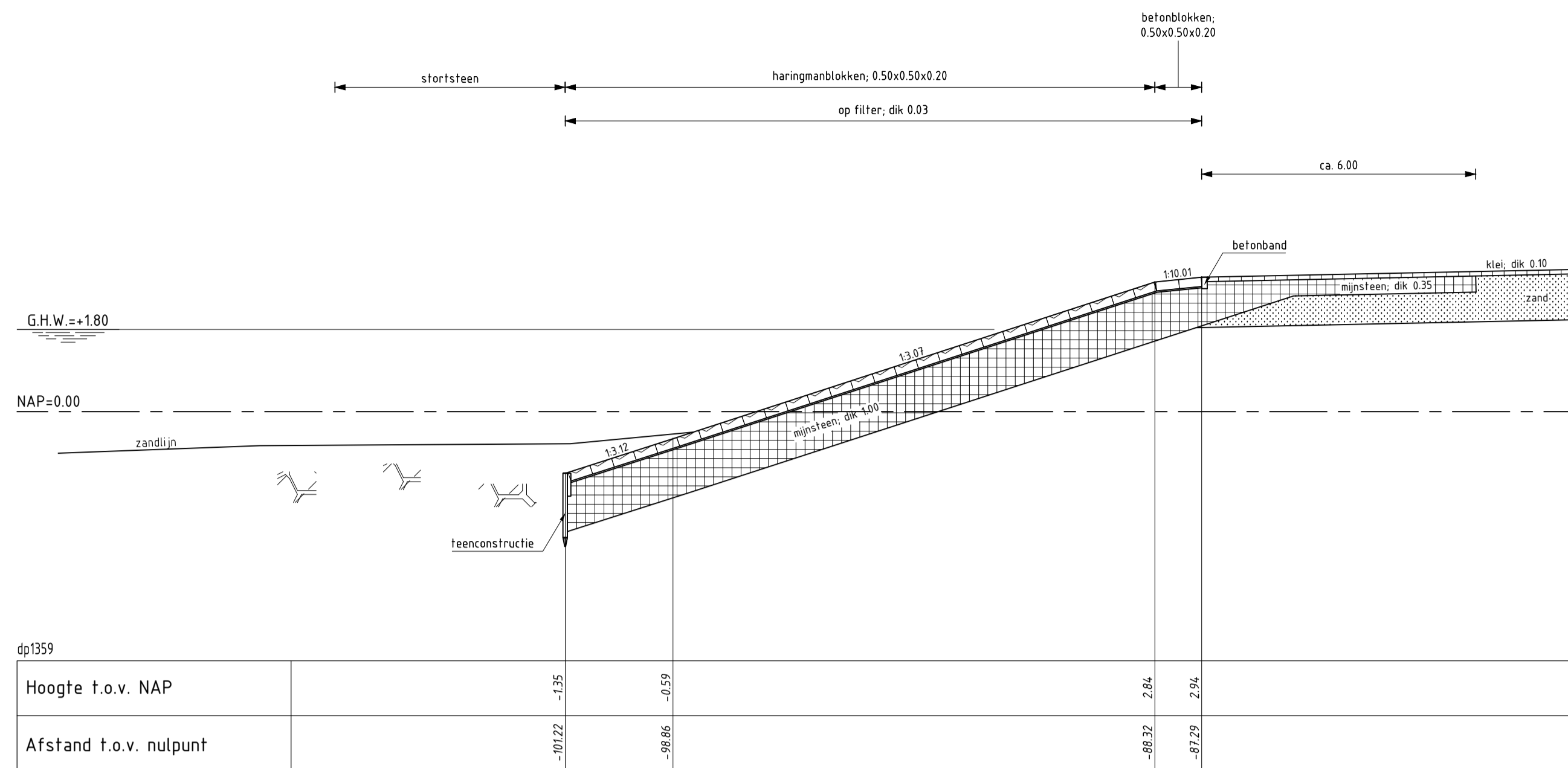
DWARSPROFIEL 1 bestaand
