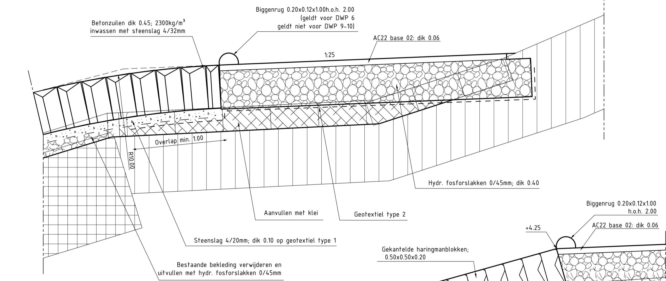
DETAIL 6 schaal 1:20
