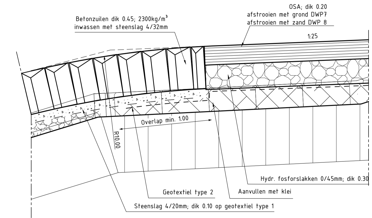
DETAIL 10 schaal 1:20
