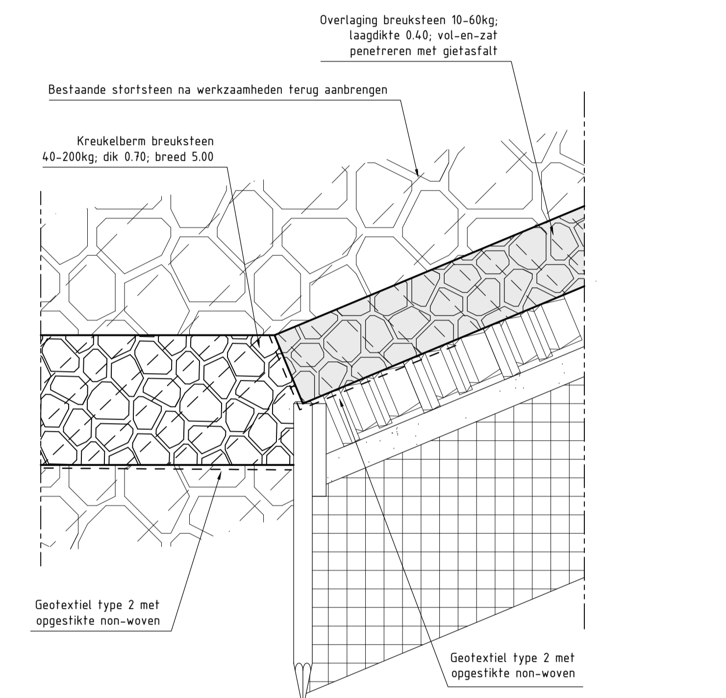
DETAIL 5 schaal 1:20
