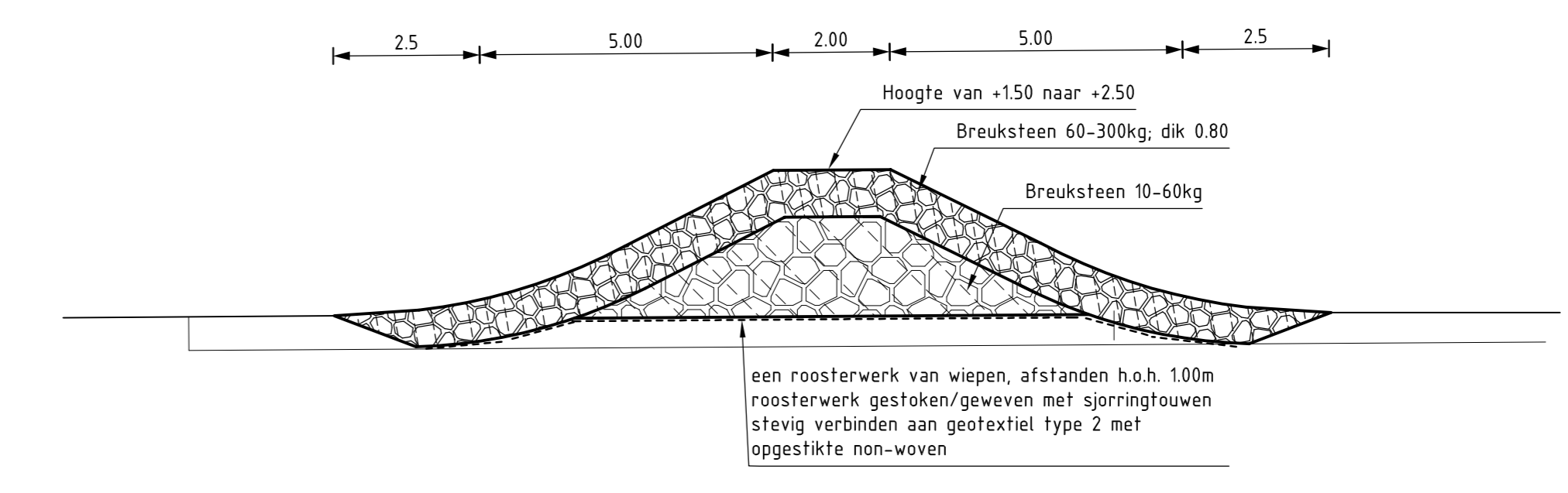
PRINCIPE DOORSNEDE "A" DAMMEN schaal 1:100
