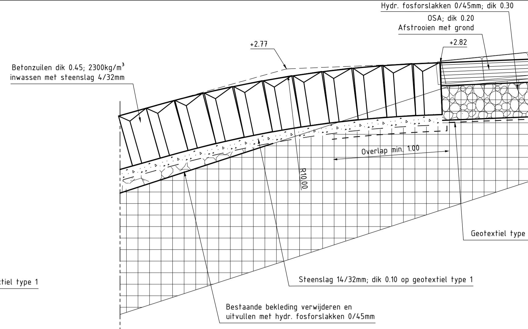
DETAIL 3 schaal 1:20
