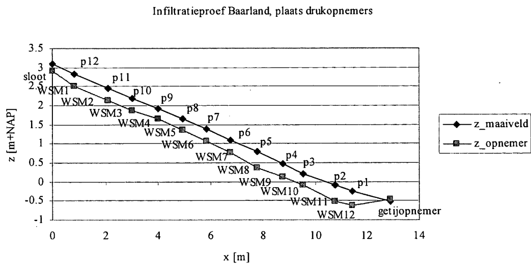
Figuur 4.2 Plaats opnemers op talud en onder talud
