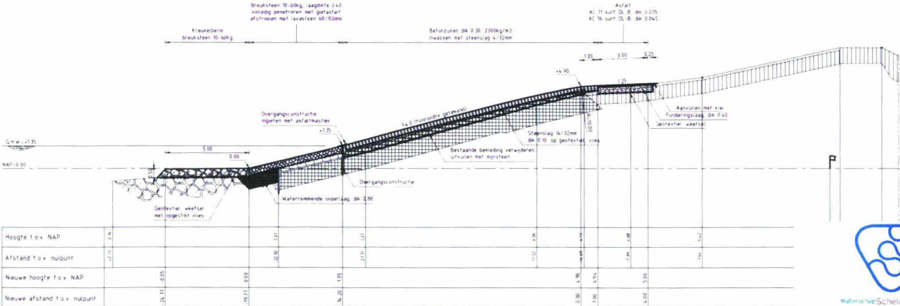
DWARSPROFIEL 5 nieuw van 01/12/2011 tot aan de laatste revisie van 11/12/2013 (zie tekening voor details) van 01/12/2011 tot aan de laatste revisie van 11/12/2013 (zie tekening voor details)
