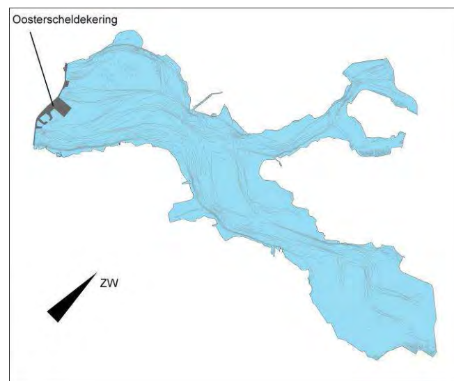
Figuur 5.10 Ligging Oosterschelde en de overheersende ZW wind- en golfrichting.
