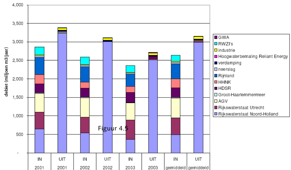
Figuur 4.6 Verdeling in- en uitdebit op jaarbasis in miljoen m 3 /jaar voor Amsterdam-Rijnkanaal en Noordzeekanaal. (bron: waterbalans Noordzeekanaal/Amsterdam-Rijnkanaal 2001-2003, RWS Noord-Holland, 2005)
