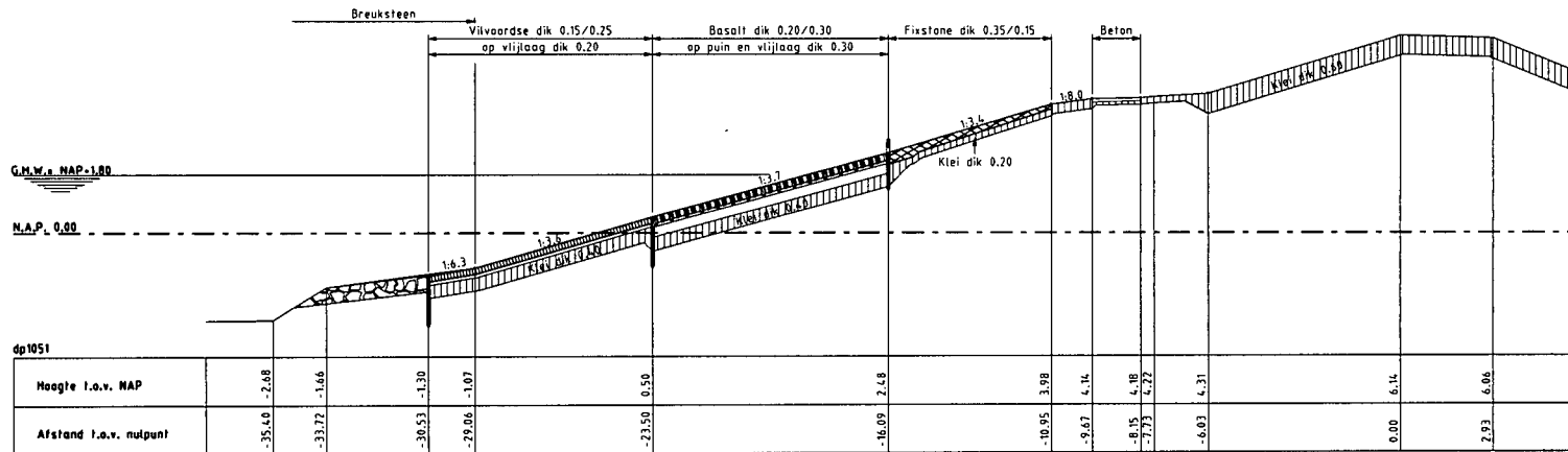
Dwarsprofiel 4 bestaand
