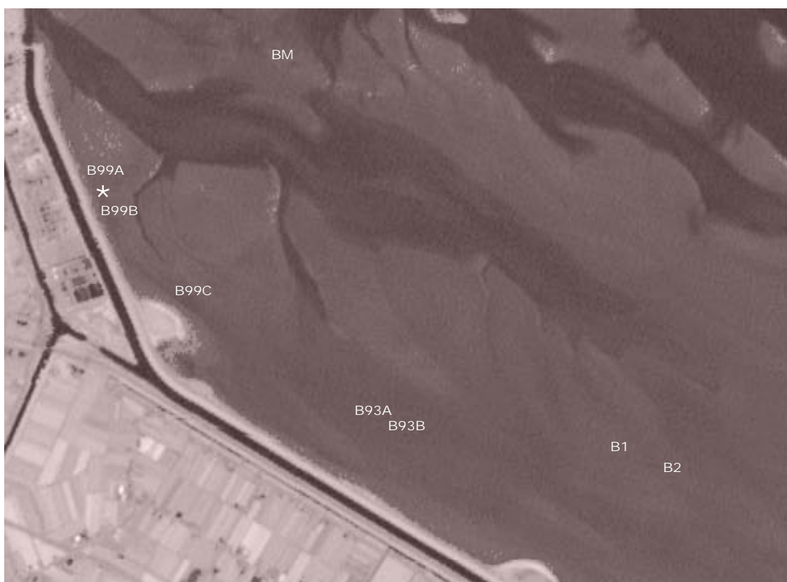
Figuur 2.1 Overzicht van de aanplantlocaties op het Balgzand. De asterisk geeft het centrum van het natuurlijke veld bij locatie B99 aan. De lichte vlekken in de knik van de dijk en aan de onderzijde van de foto representeren het Kooyhoekschor en het Van Ewijkksluisschor. Bron: Landsat.
