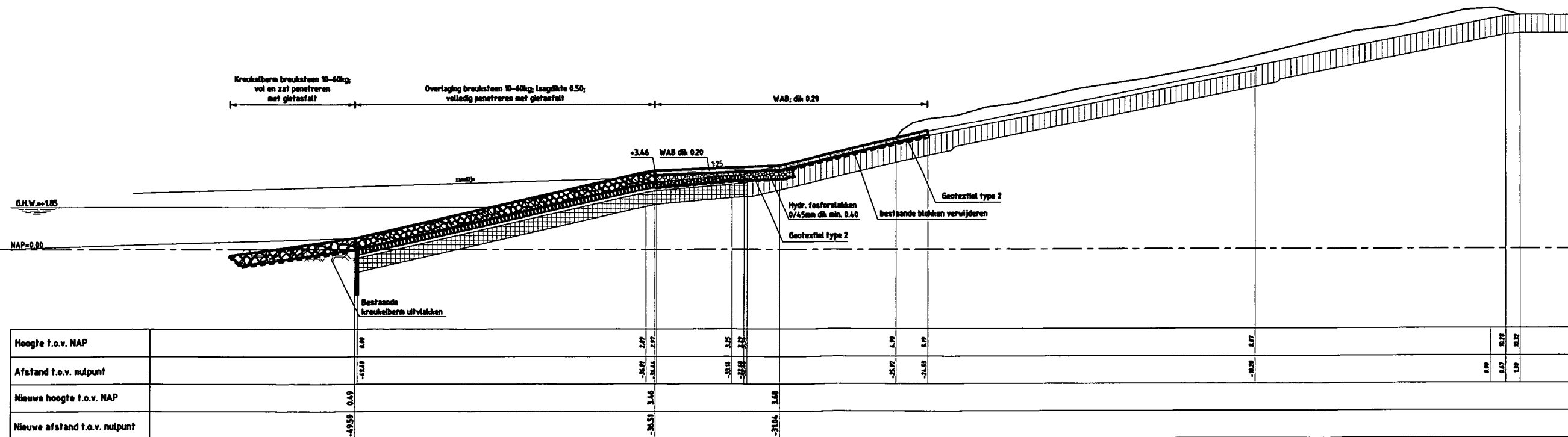
DWARSPROFIEL 1 nieuw van dp211 tot dp214 +12m schaal 1:100
