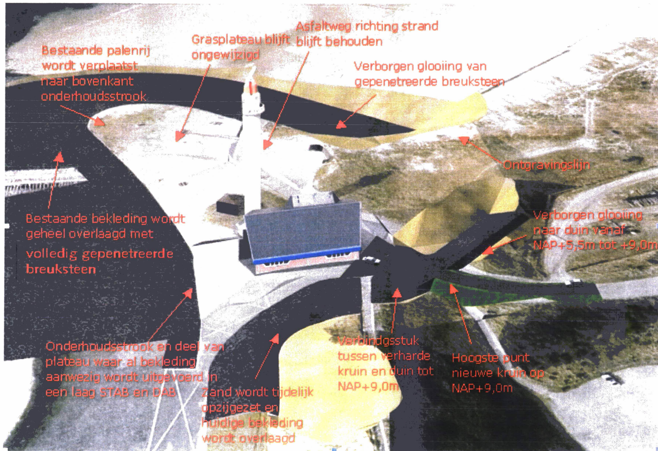
Figuur 13a: Bovenanzicht nieuwe situatie plateau Zuiderdam 3D
