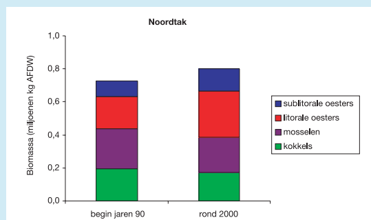
Figuur 7.5 De biomassa van kokkels, mosselen en oesters in de Noordtak van de Oosterschelde begin jaren negentig en rond 2000.
