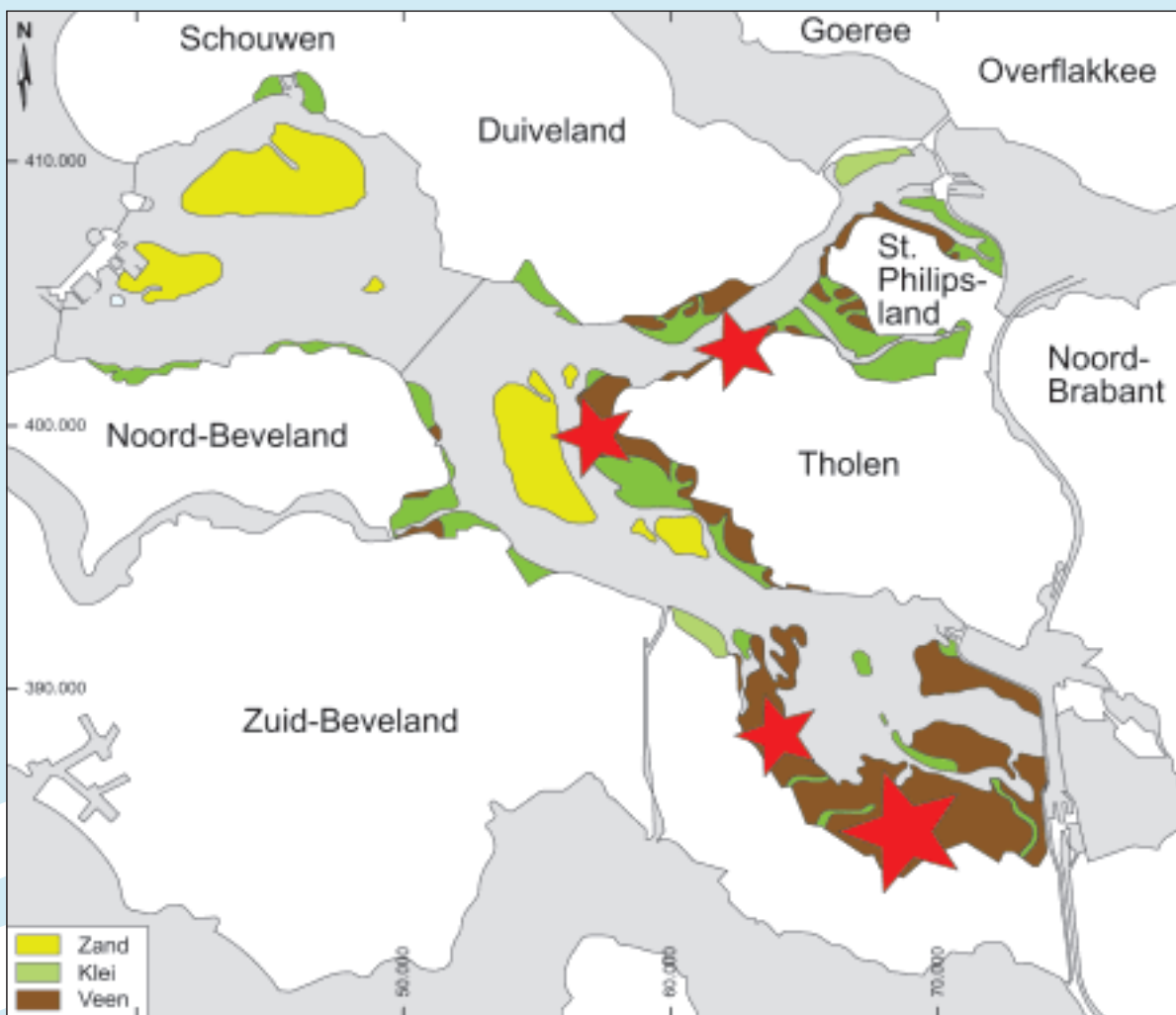
Figuur 2.10 Het voorkomen van veen in de ondergrond van Zeeland. Met een rode ster is aangegeven waar veen dagzomend (Naar Fischer, 1997).
