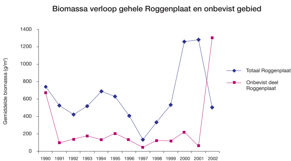
Figuur 5.23 Verloop van de gemiddelde kokkelbiomassa's (g/m² versgewicht) op de gehele Roggenplaat en in het voor kokkelvisserij gesloten gebied per jaar.
