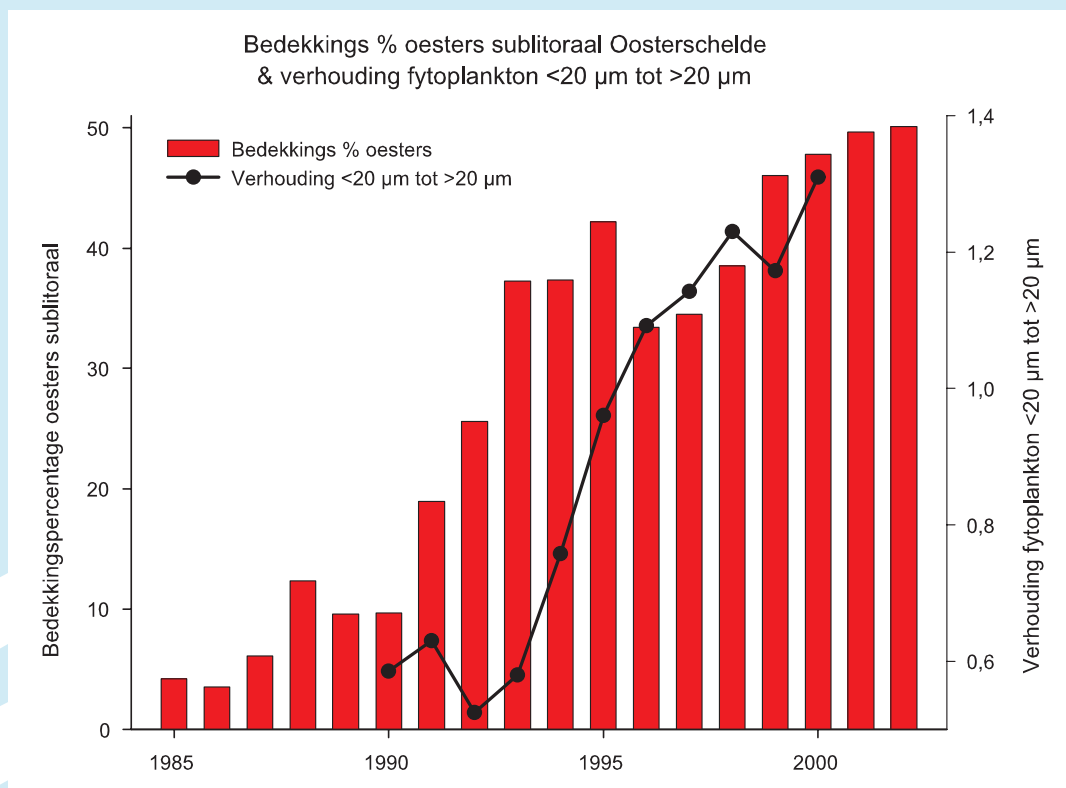
Figuur 7.9 Verhouding fytoplankton <20 µm tot >20 µm (zwarte lijn) en het bedekkingspercentage met Japanse oesters (gegevens AquaSense) gemiddeld voor de gehele Oosterschelde ( r^2 = 0,71 , p < 0,01 ).
