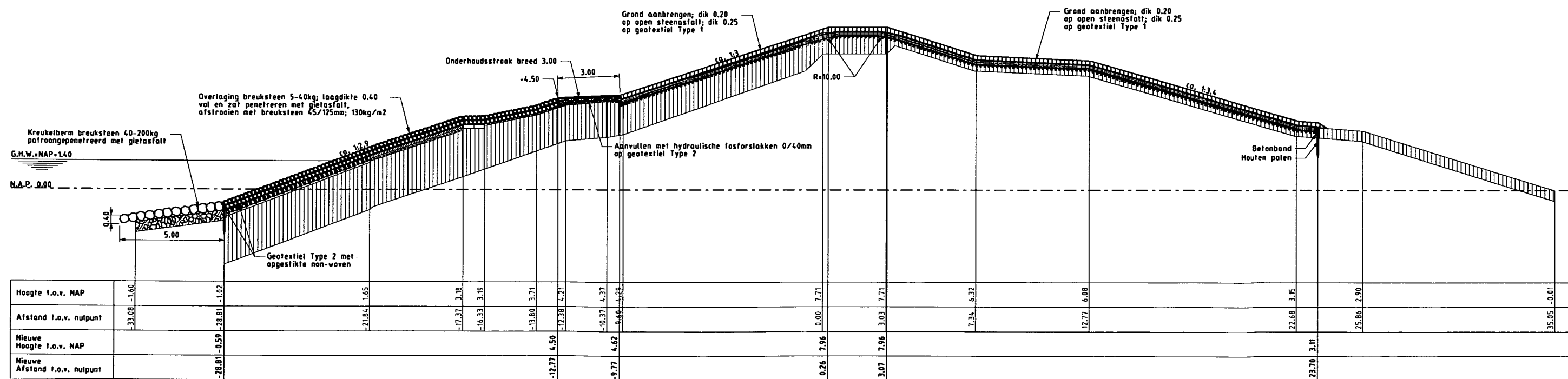
Dwarsprofiel 2 nieuw
