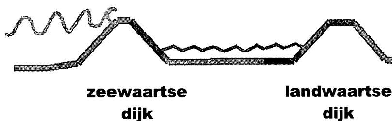
Figuur 2.1 Waterkeringstelsel tussen dp 148+50m en dp 160
