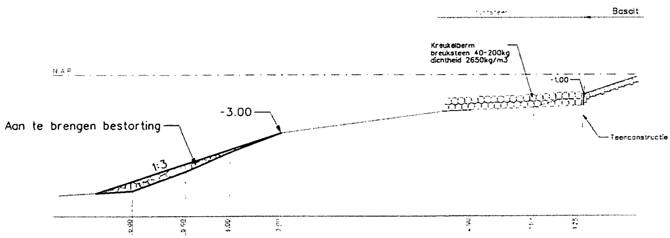
Dwarsprofiel Schaal 1:200
