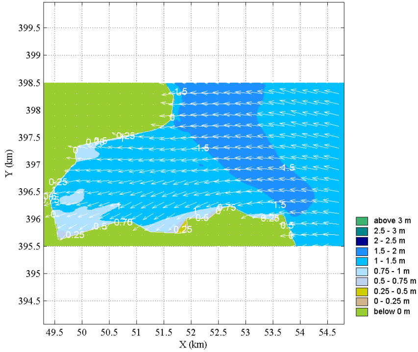
Grid: D07, Wind 90°, Hoog water, 4 m +NAP windsnelheidsklasse 2
