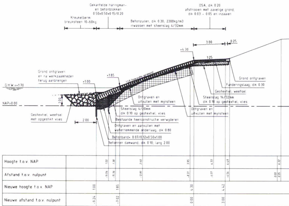
DWARSPROFIEL 4a nieuw
