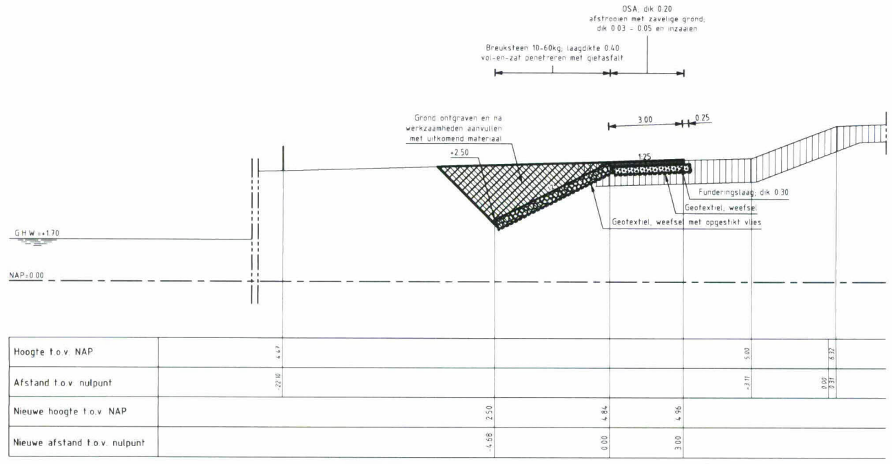
DWARSPROFIEL 3 nieuw van dp714+49m tot dp717+46m
