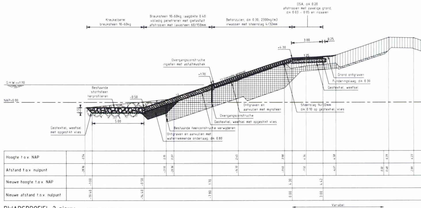
DWARSPROFIEL 2 nieuw van dp714+50m tot dp714+49m
